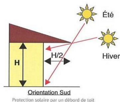
Orientation Sud
