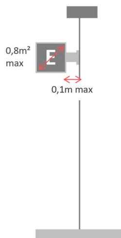
Schématisation de la règle relative aux enseignes perpendiculaires (schéma indicatif et non opposable)
