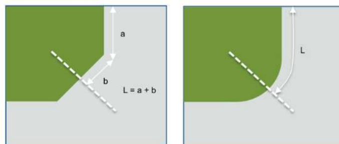
Schématisme de la règle de calcul de la densité dans le cas particulier d'un pan coupé (schéma indicatif et non opposable)
