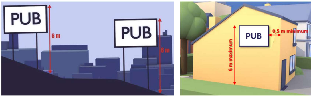
Schématisation de la règle de hauteur pour les dispositifs scellés au sol ou installés directement sur le sol et pour les dispositifs muraux (schéma indicatif et non opposable)
