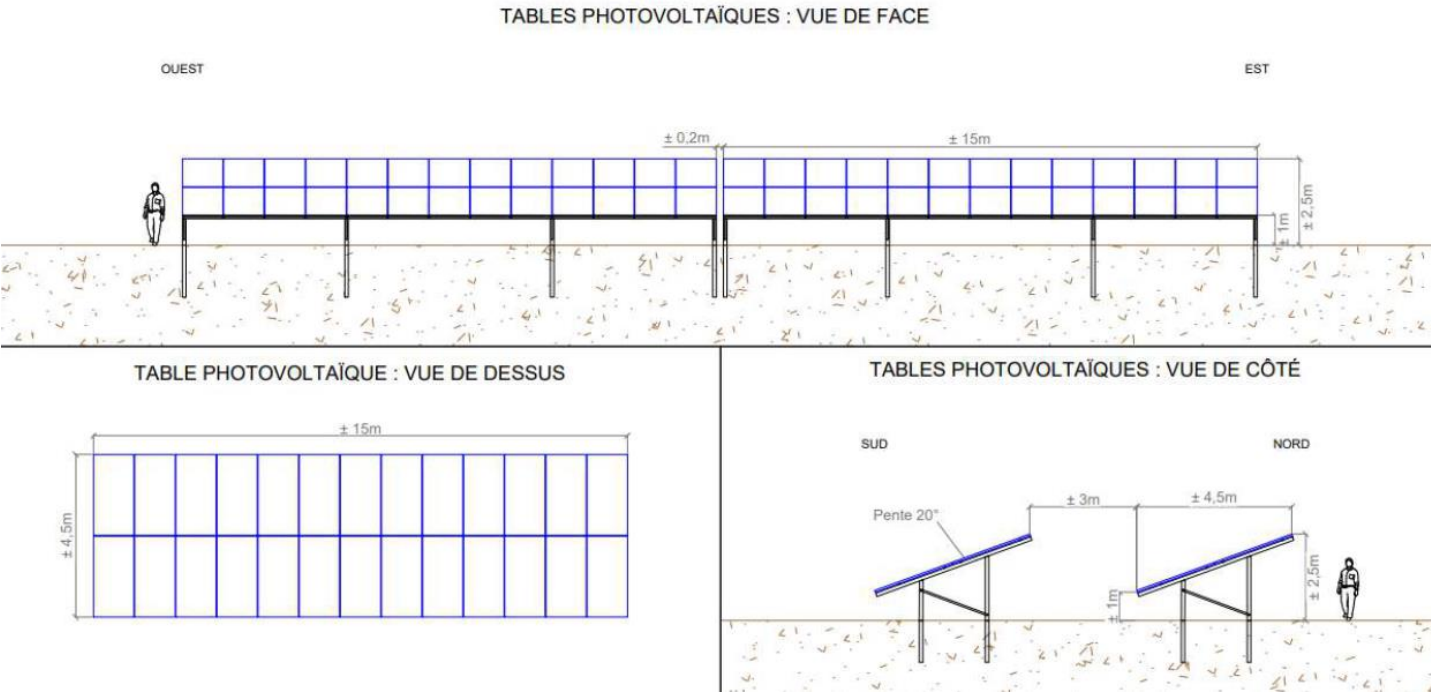
Illustration 15 : Coupe de structures photovoltaïques fixes sur pieux Source : TotalEnergies Renouvelables France, 2023
