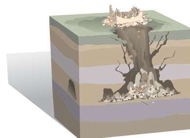
Propagation du vide vers la surface
