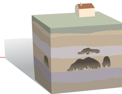
Cavité naturelle ou artificielle
