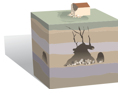
Effondrement de la cavité
