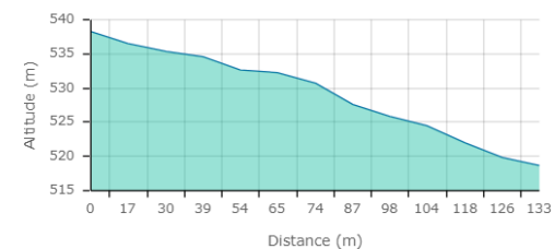
PROFIL ALTIMÉTRIQUE
