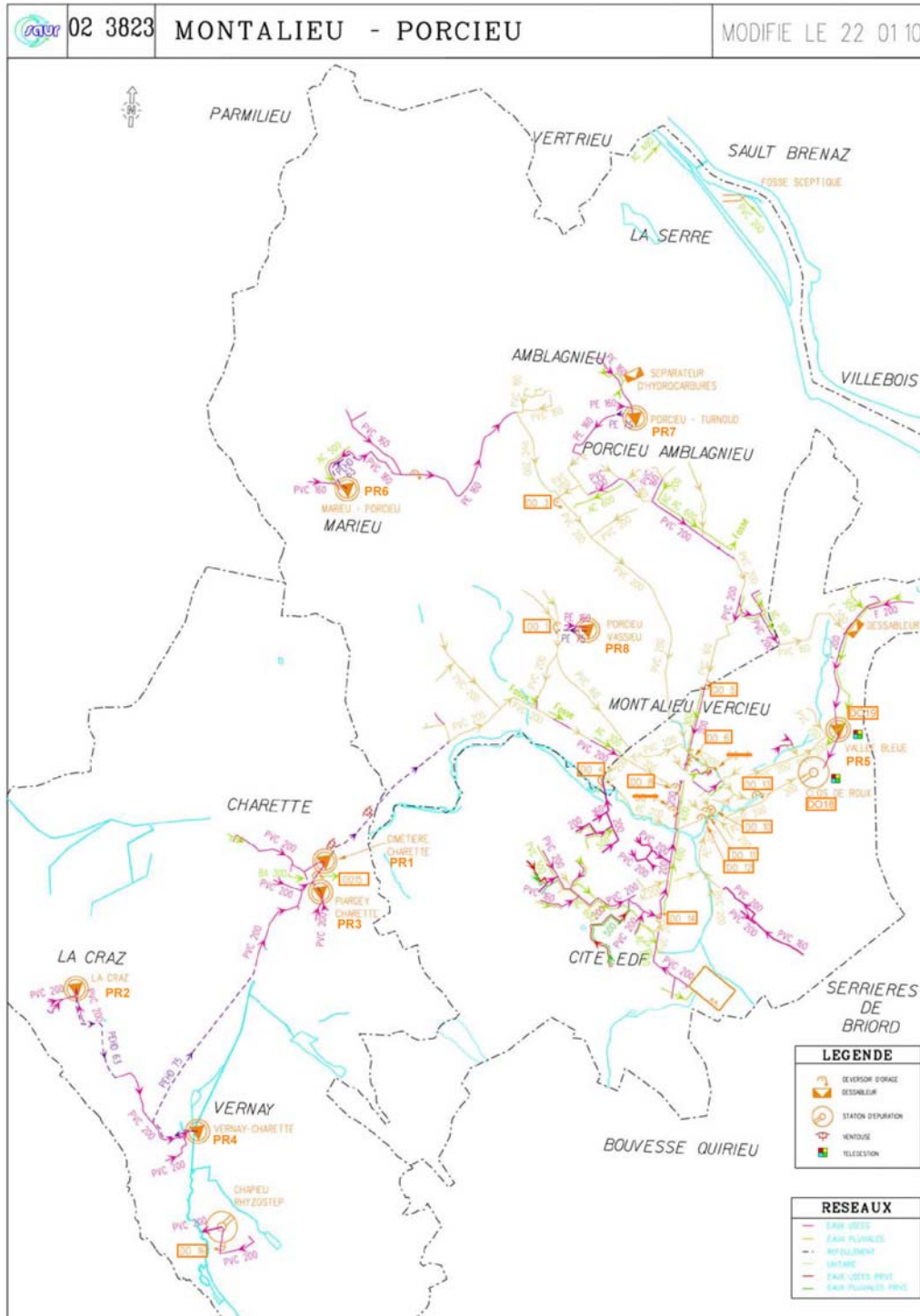
Figure 9 : Localisation déversoirs d'orage et trop plein
