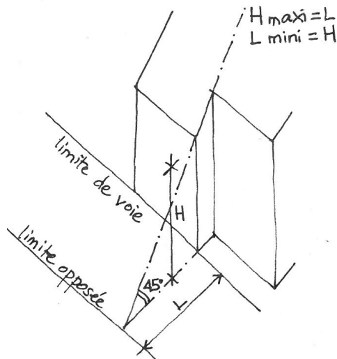
Schéma 1 – Implantation en limite d'emprise publique ou de voie (prospect à 45^\circ ) L . supérieure ou égale à H
