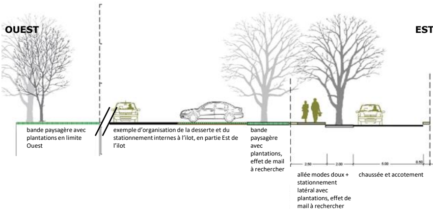
Principe de profil en travers de la voie A et ses abords
