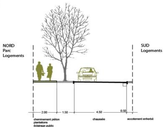
Principe de profil en travers de la voie à créer et ses abords
