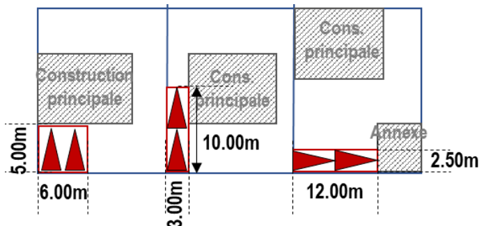
Propositions d'implantation des aires de stationnement pour les constructions à usage d'habitation.
