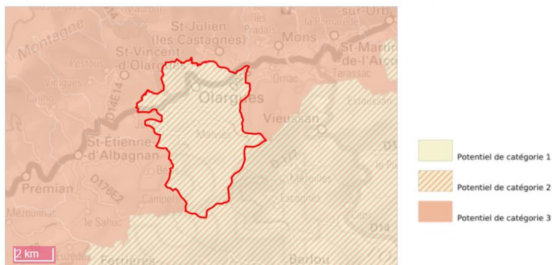
CARTOGRAPHIE 19 : RISQUES LIE AU RADON - SOURCE BRGM
