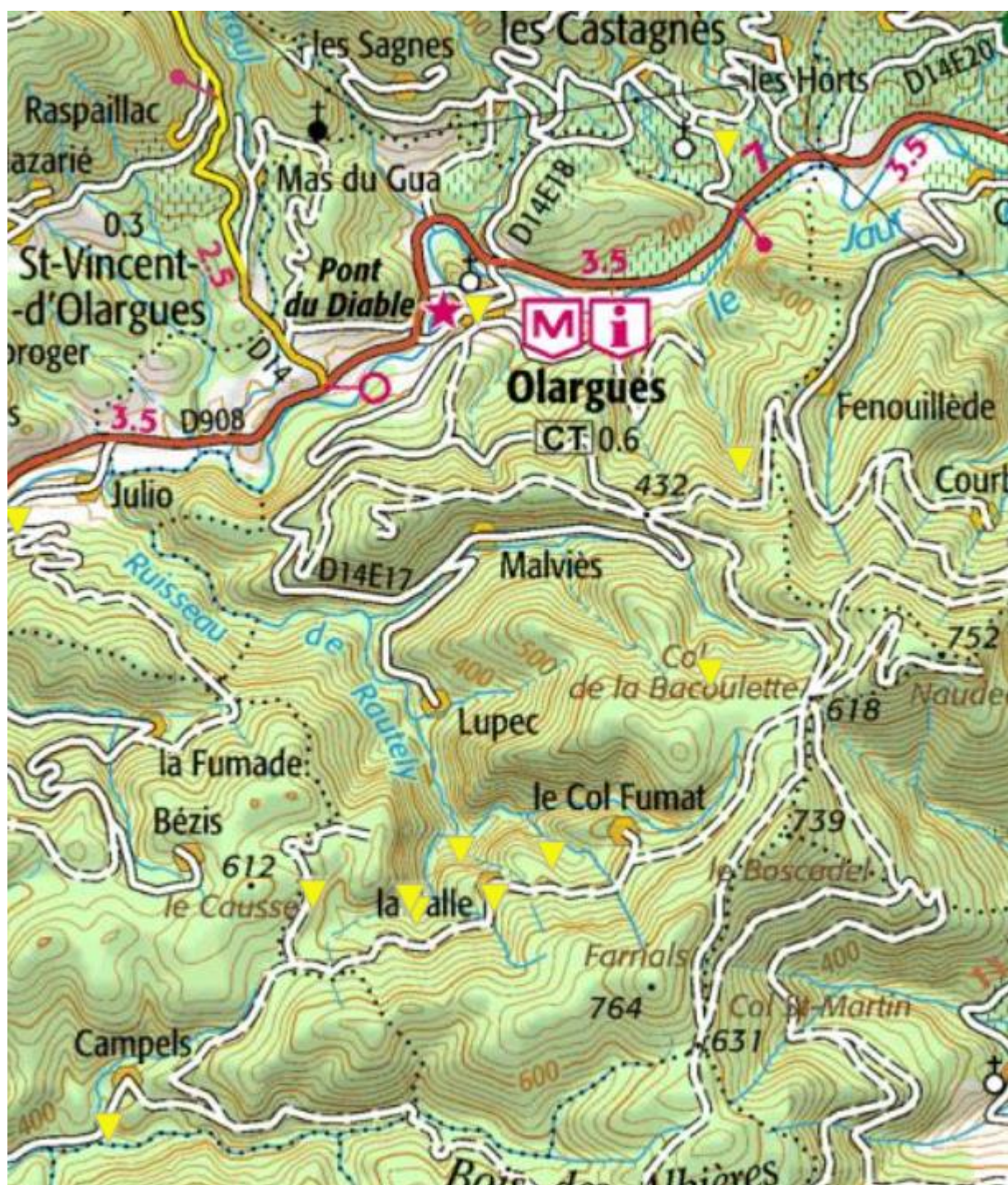
CARTOGRAPHIE 16 : PRESENCE DE CAVITES - SOURCE BRGM
