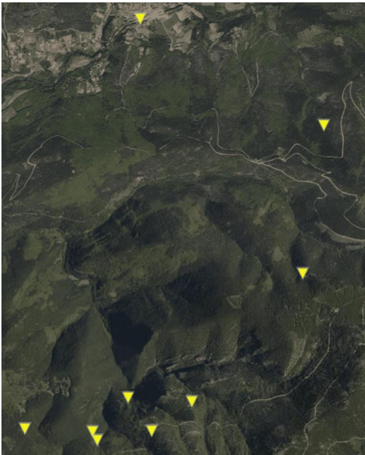
CARTOGRAPHIE 17 : PRESENCE DE CAVITES - SOURCE BRGM
