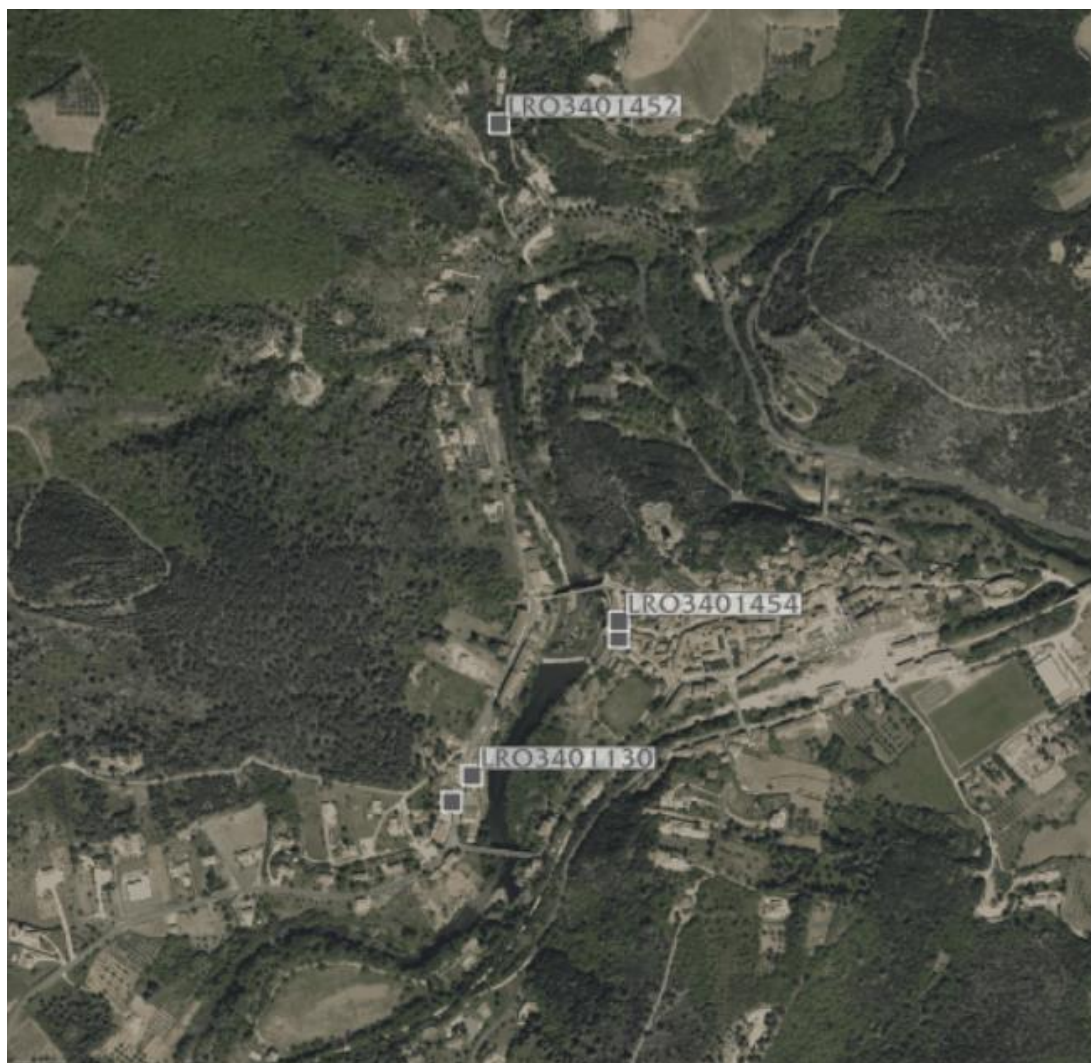
CARTOGRAPHIE 18 : PRESENCE DE CAVITES - SOURCE BRGM
