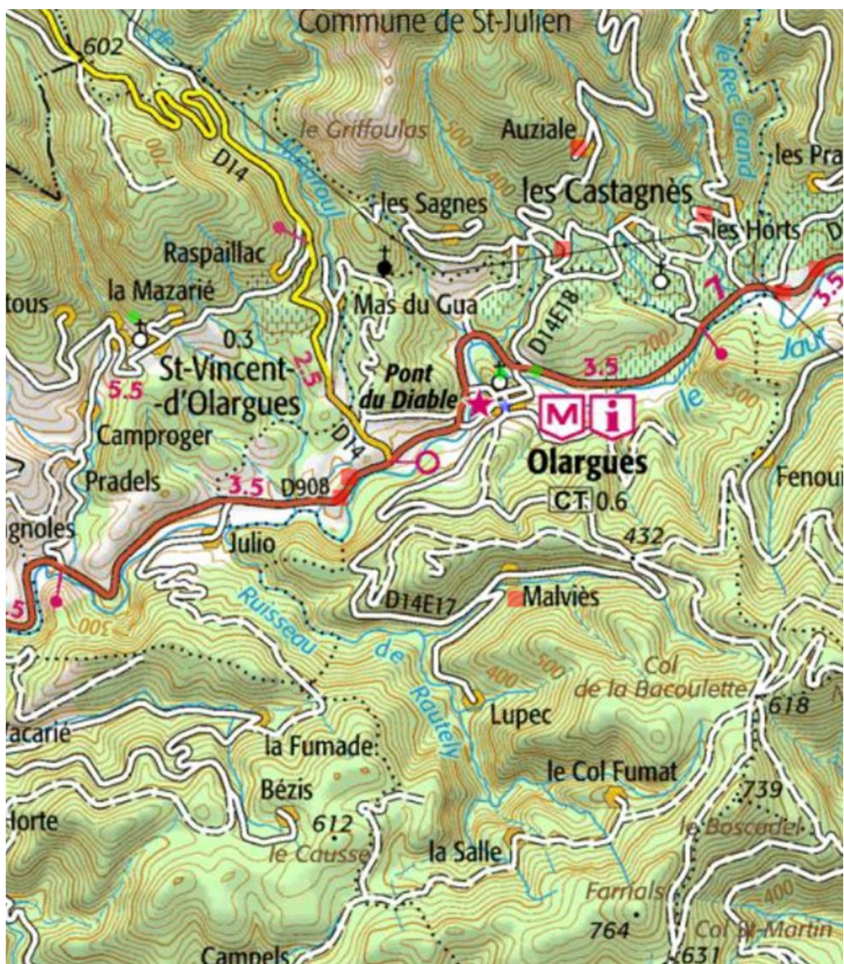
CARTOGRAPHIE 12 : RISQUES DE MOUVEMENT DE TERRAIN - SOURCE BRGM
