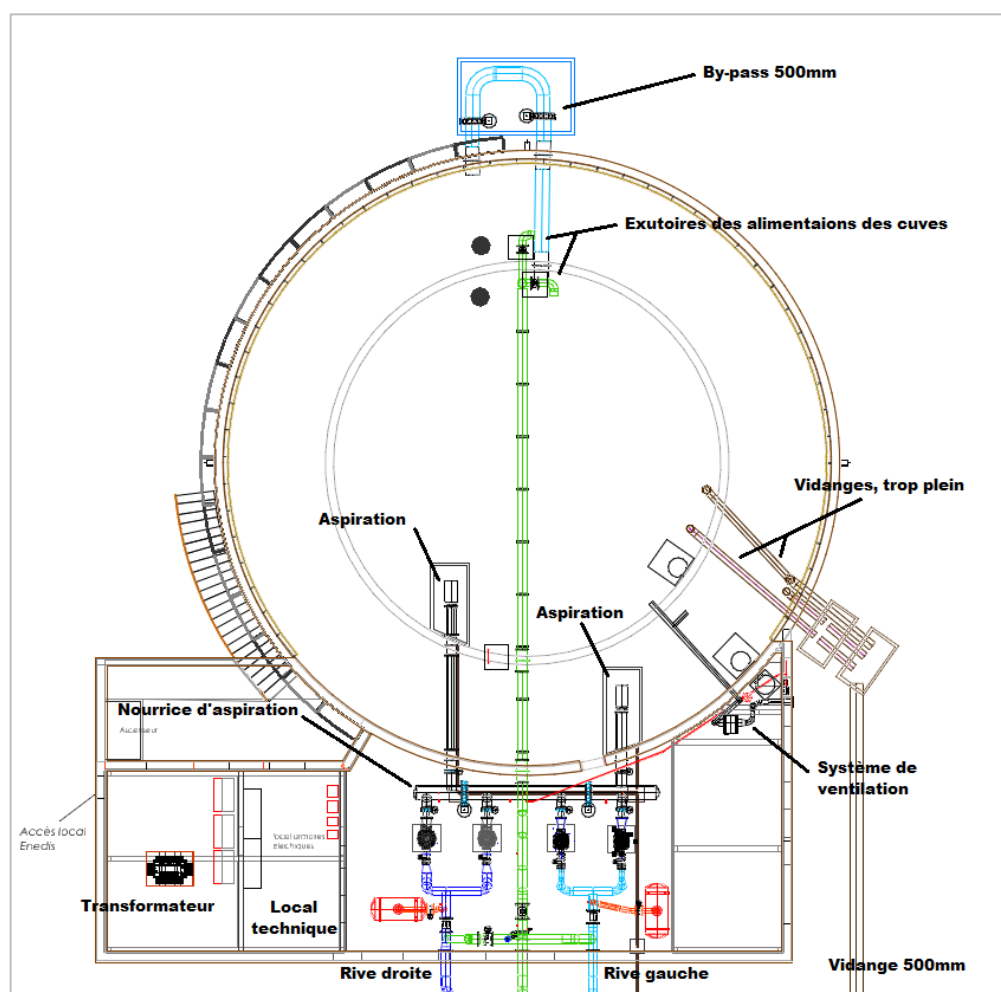
Figure 5 - Schéma général de la nouvelle station de Cazouls - Source bureau d'études SMEVH
