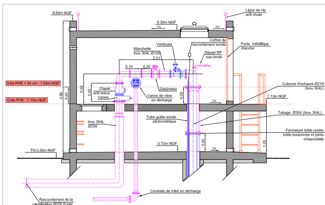
Figure 4 - Exemple de schéma de principe d'un aménagement
