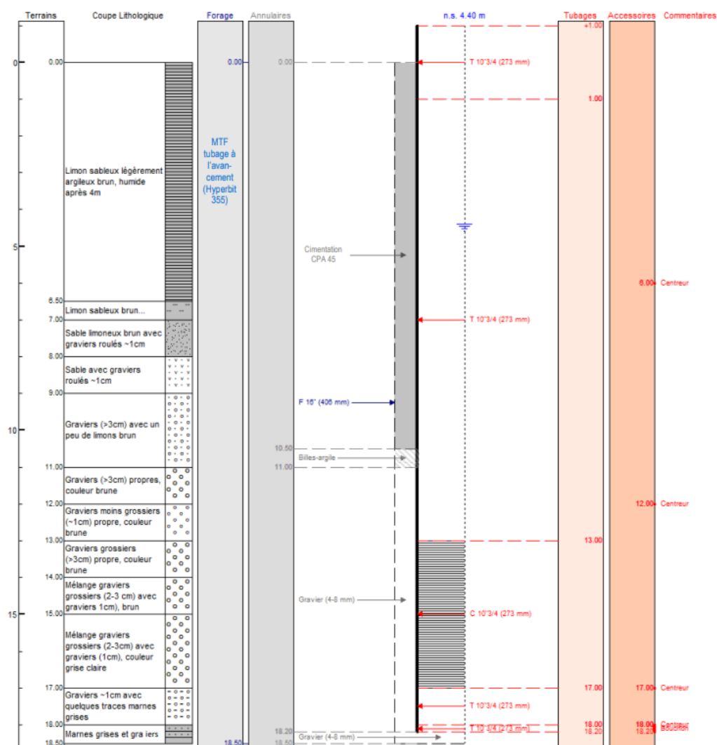
Figure 6 - Coupe géologique et technique du nouveau forage FR1-2023
