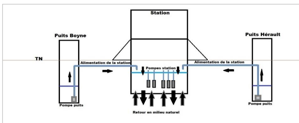
Figure 2 - Schéma de principe du fonctionnement de la bache
