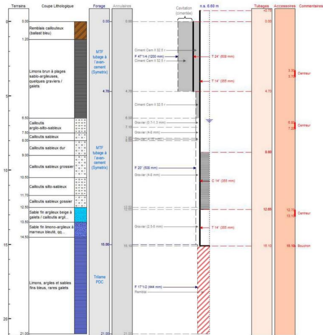
Figure 4 - Coupe géologique et technique du nouveau forage FR-2020
