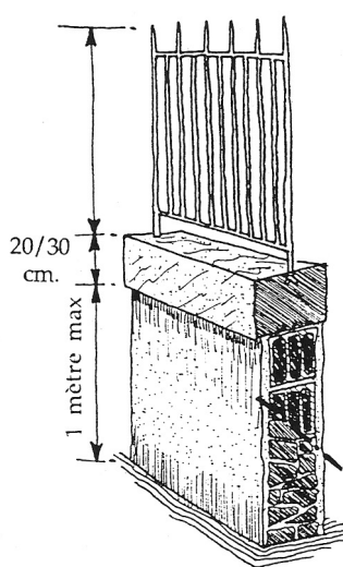
MUR-BAHUT ET BARREAUDAGES
