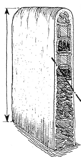
CLÔTURE À GLACIS.
