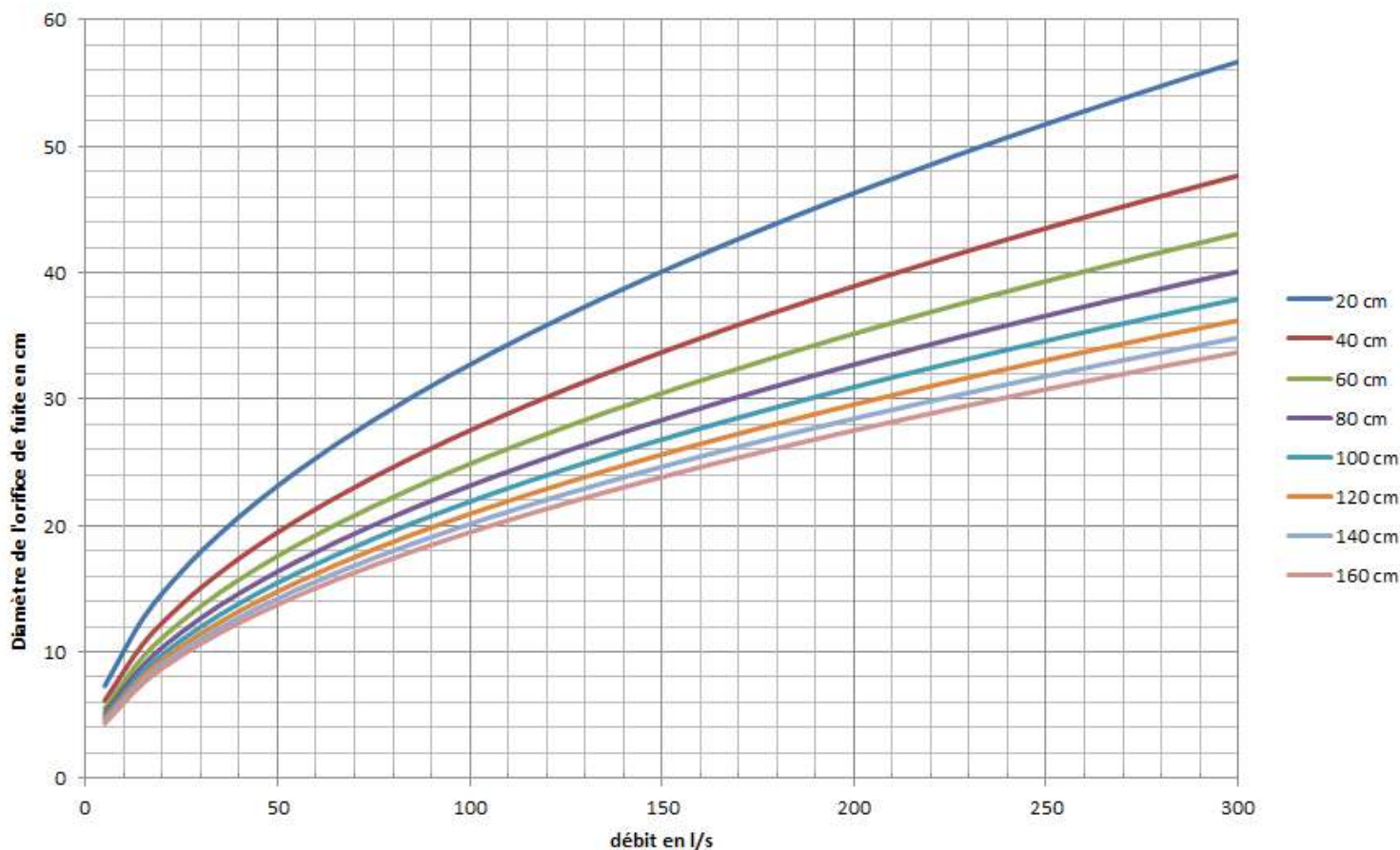
ABQUES POUR LE DIMENSIONNEMENT DES ORIFICES DE R GULATION
