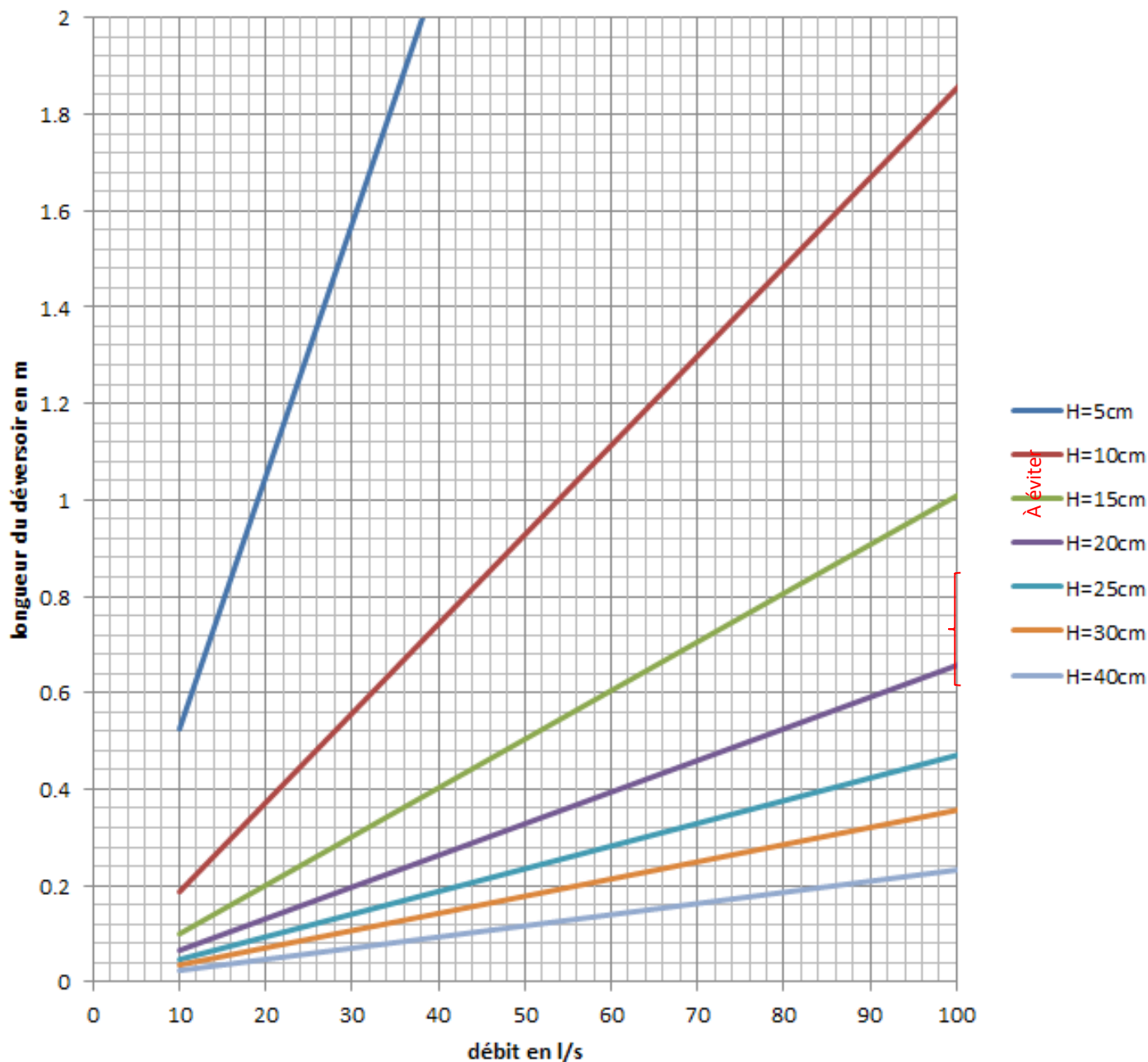
ABaque 1 GAMME DE D BIT DE 1 L/S - D VERSOIR RECTANGULAIRE SEUIL PAIS D NOY
