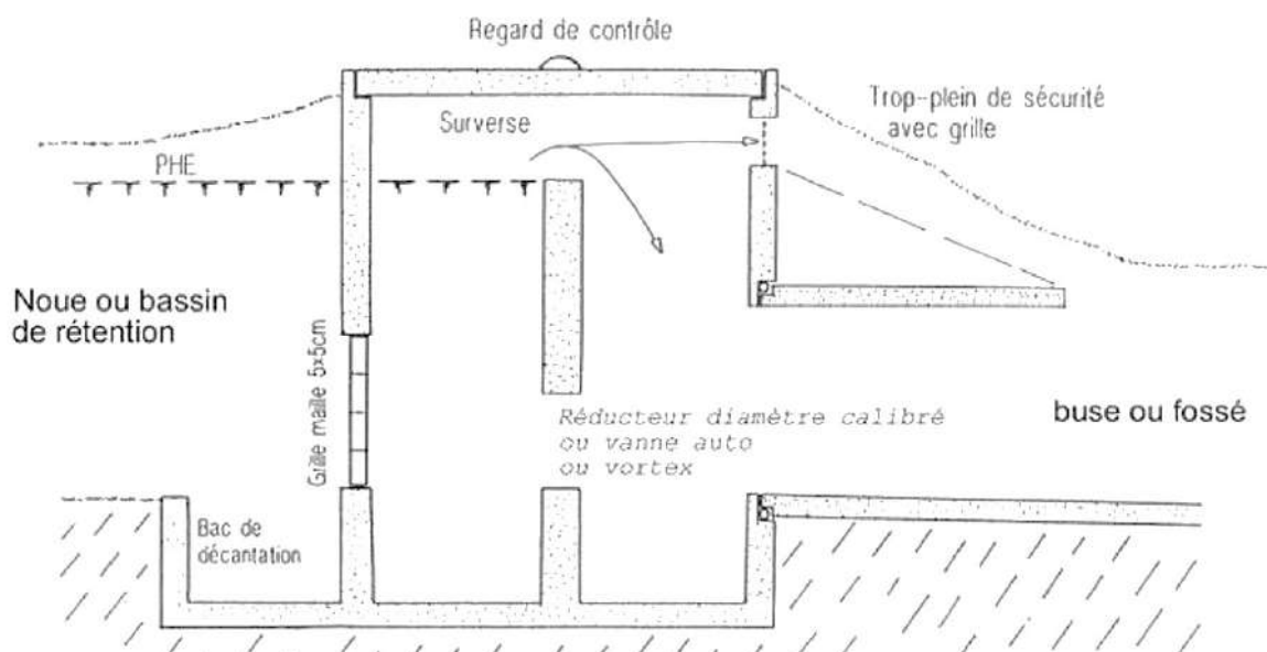
PETIT OUVRAGE EN B TON AVEC ORIFICE ET SURVERSE INT GR
