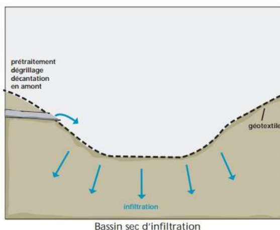
PRINCIPES DES BASSINS DE RÉTENTION SEC / EN EAU (SOURCE GRAIE)
