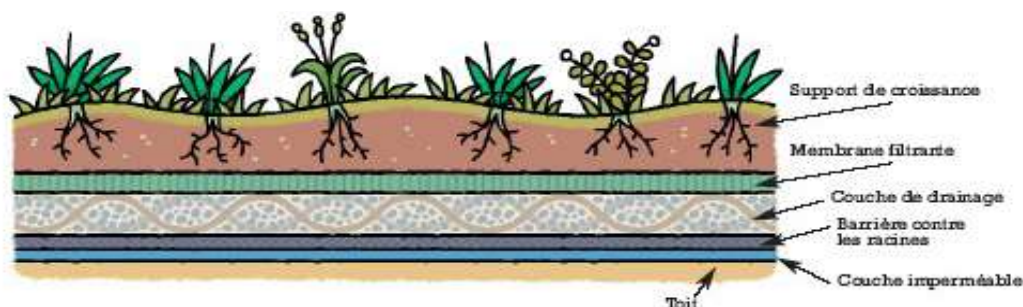
COUPE D'UN TOIT V G TALIS (SOURCE GRAND LYON)
