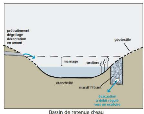
PRINCIPES DES BASSINS DE RÉTENTION SEC / EN EAU (SOURCE GRAIE)
