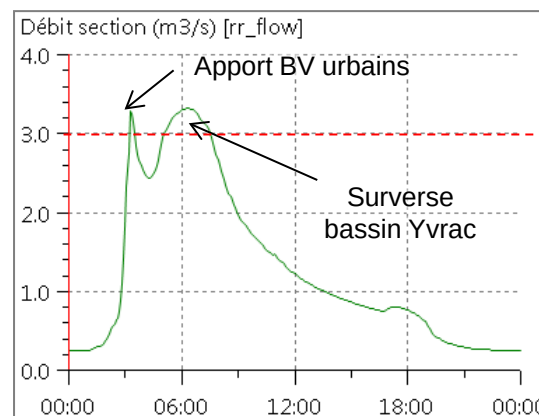
Hydrogramme Georges Bizet – T = 100 ans
