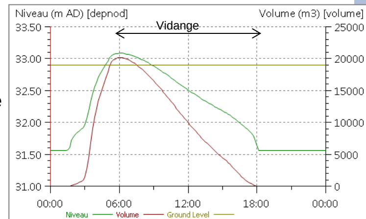
Situation de référence - T = 20 ans
