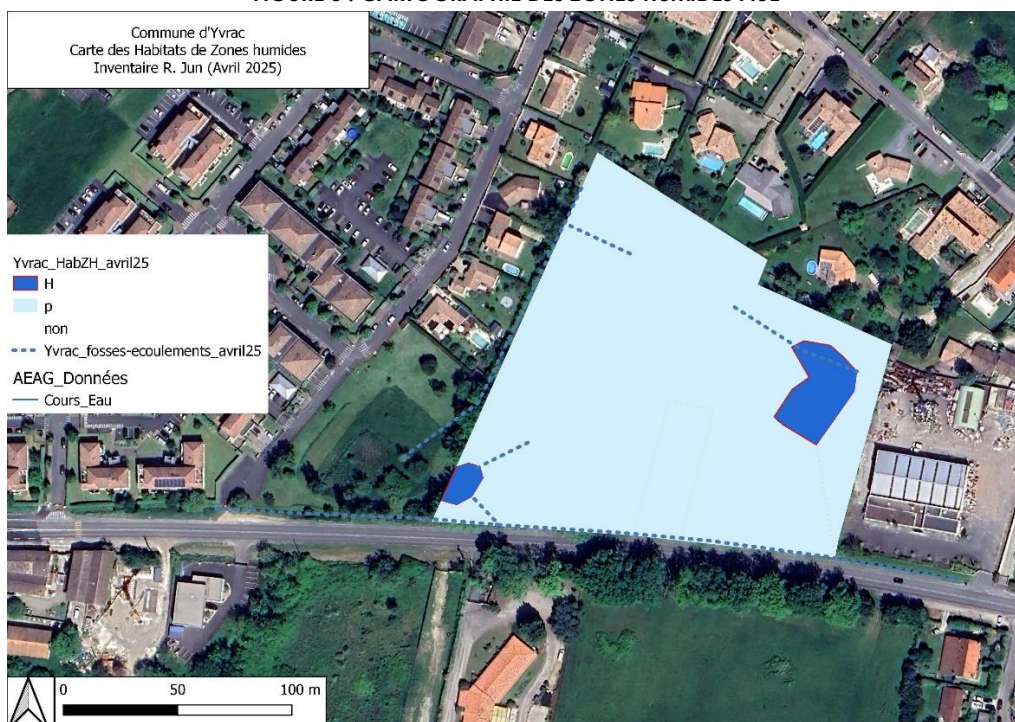
FIGURE 5 : CARTOGRAPHIE DES ZONES HUMIDES AUE
