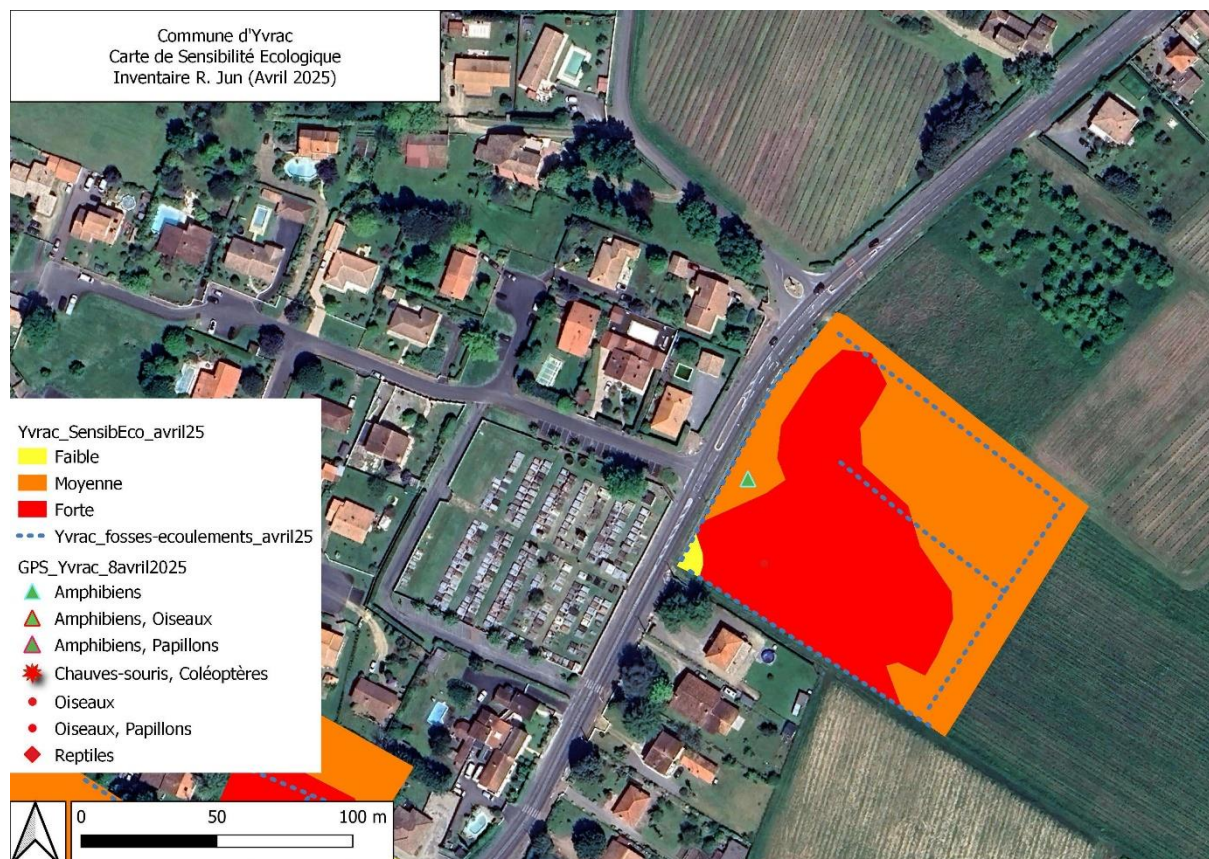
FIGURE 16 : CARTOGRAPHIE DES ENJEUX ECOLOGIQUES SUR ER n°12
