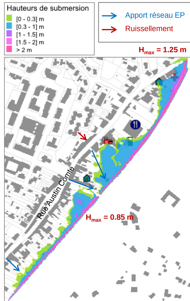
Emprise de la zone inondable – simulation de la pluie du 26/07/2013
