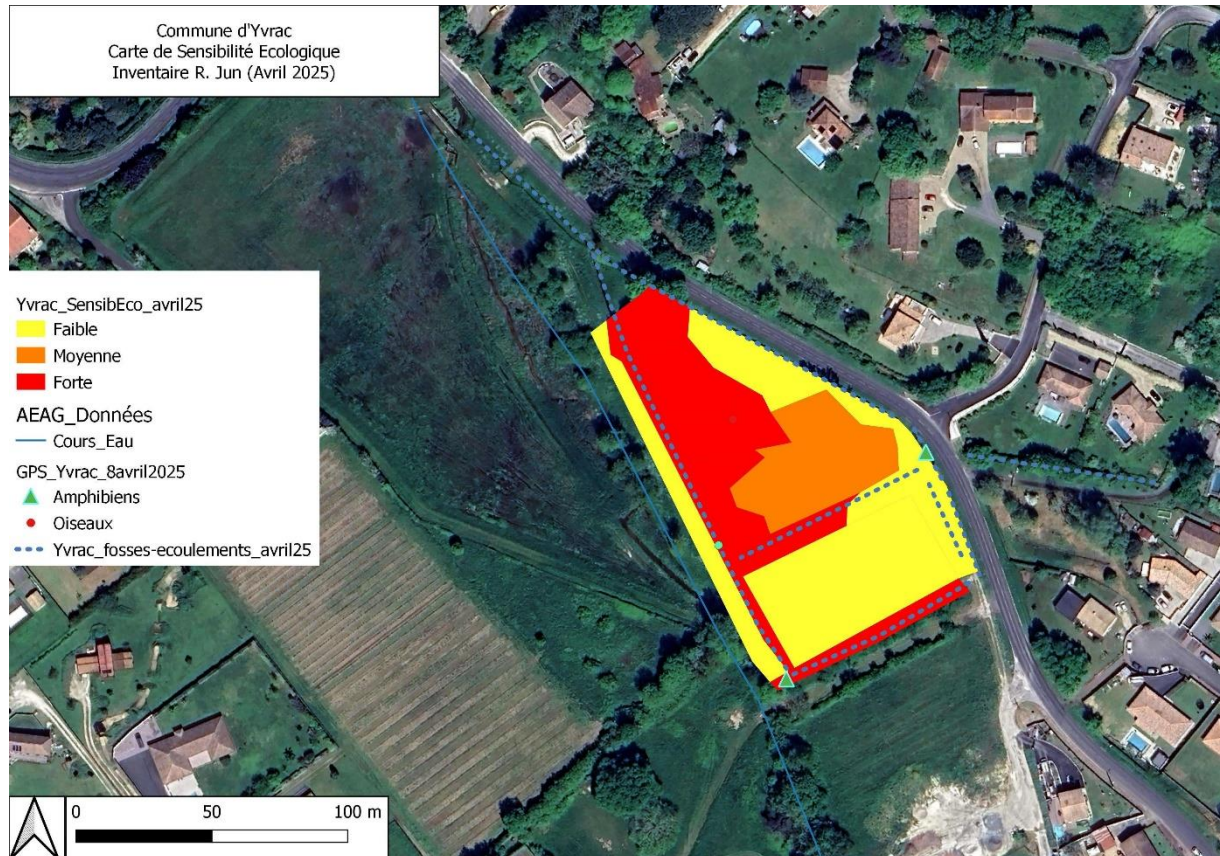
FIGURE 14 : CARTOGRAPHIE DES ENJEUX ECOLOGIQUES SUR ER n°4
