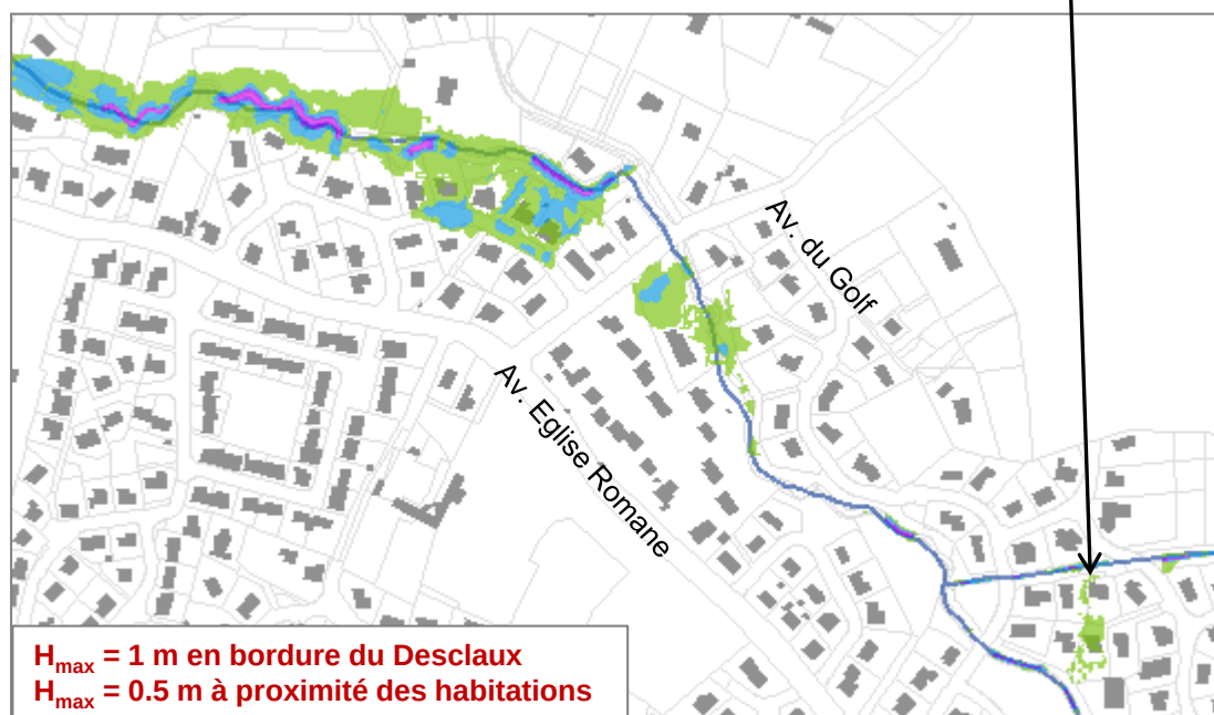
Emprise de la zone inondable – simulation de la pluie du 26/07/2013
