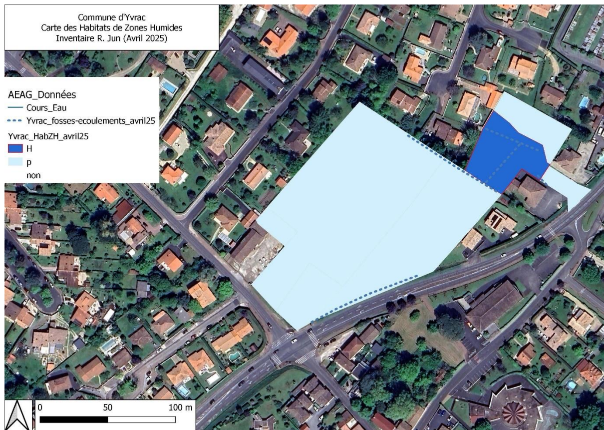
FIGURE 3 : CARTOGRAPHIE DES HABITATS DE ZONES HUMIDES AUa/b
