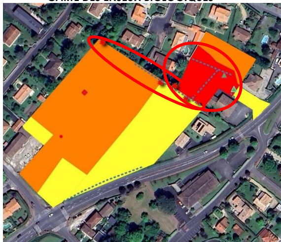
CARTE DES ENJEUX BIOLOGIQUES
