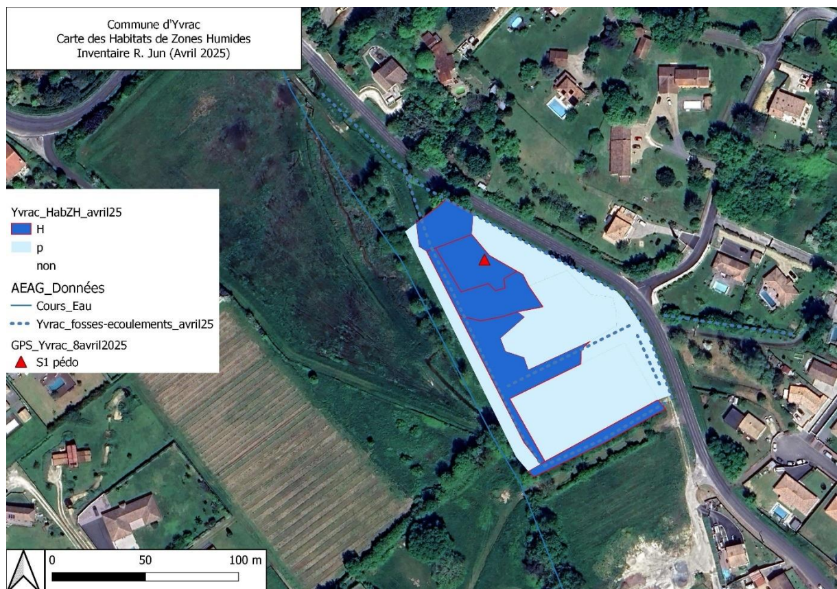
FIGURE 7 : CARTOGRAPHIE DES SONDAGES PEDOLOGIQUES ET ZONES HUMIDES - ER4 (typologie Corine Biotopes)
