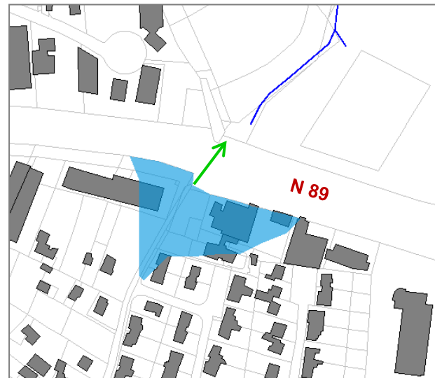
Zone inondable du 26/07/2013
