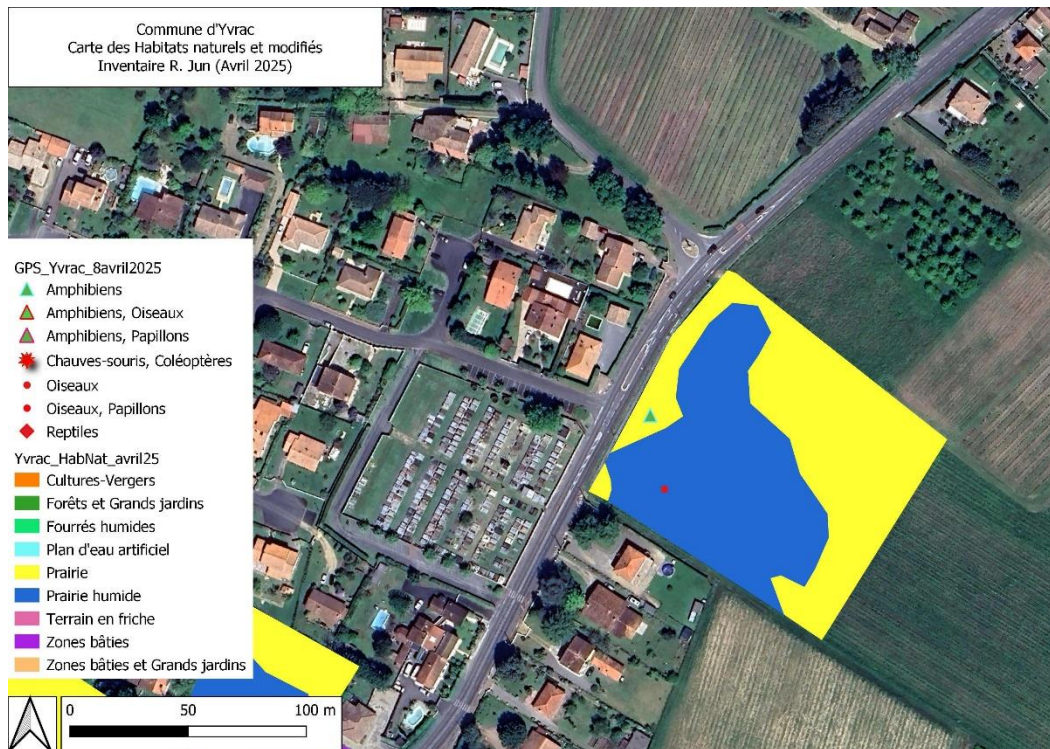
FIGURE 10 : CARTOGRAPHIE DES HABITATS NATURELS ET MODIFIEES ER12 (typologie Corine Biotopes)
