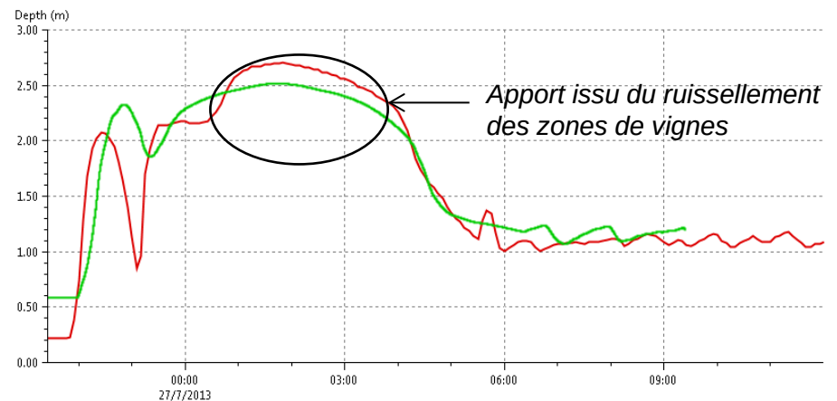
Exemple : Hauteur d'eau dans le Gua (Archeveque aval)
