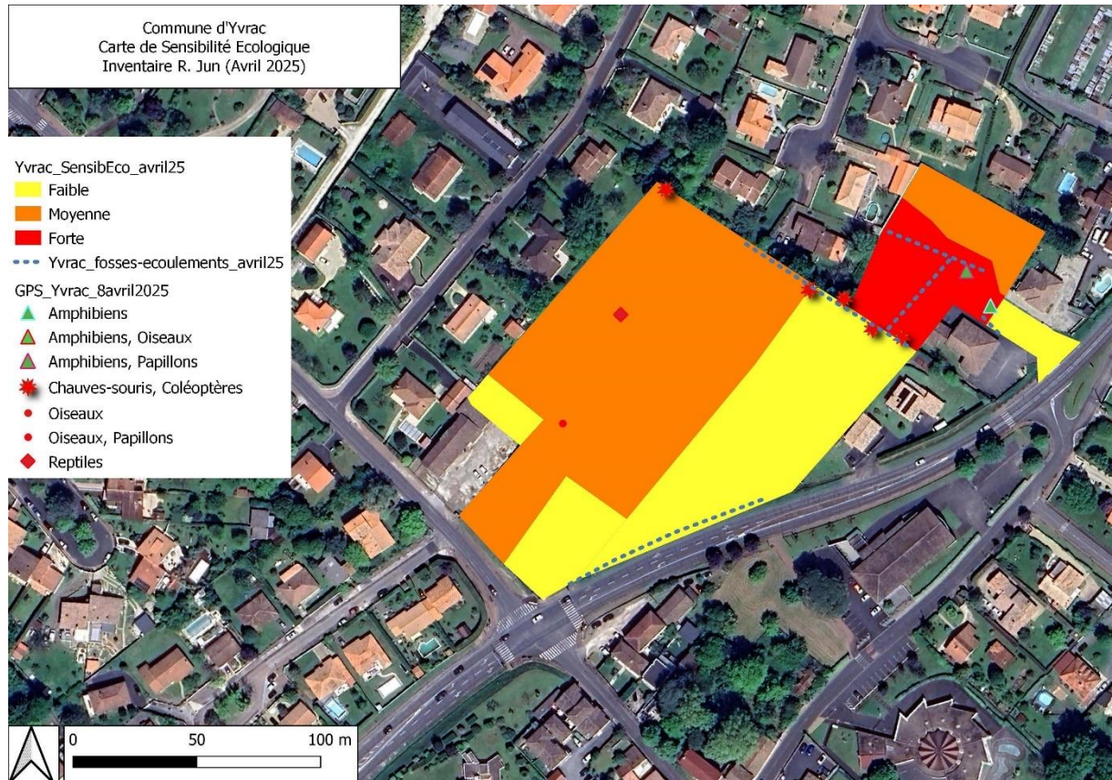
FIGURE 12 : CARTOGRAPHIE DES ENJEUX ECOLOGIQUES SUR LES SECTEURS AUa/b
