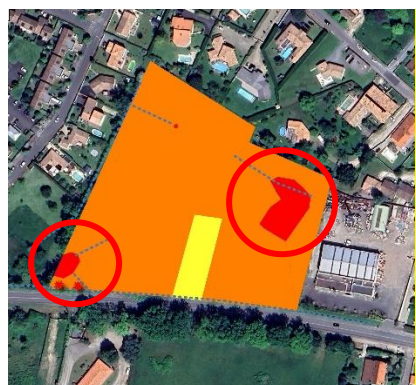
CARTE DES ENJEUX BIOLOGIQUES
