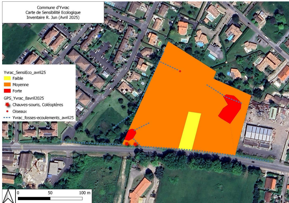
FIGURE 13 : CARTOGRAPHIE DES ENJEUX ECOLOGIQUES SUR LE SECTEUR AUE Route du Périgord
