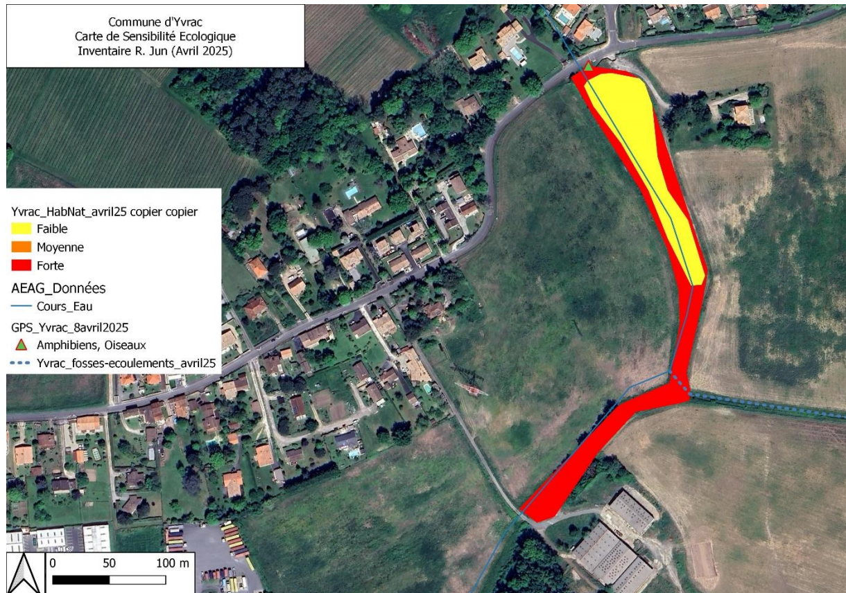
FIGURE 15 : CARTOGRAPHIE DES ENJEUX ECOLOGIQUES SUR ER n°5
