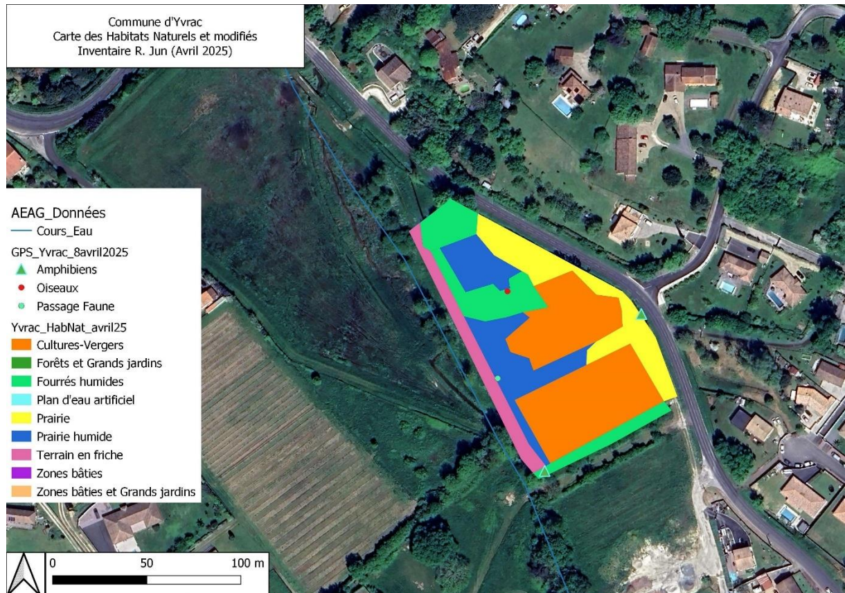
FIGURE 6 : CARTOGRAPHIE DES HABITATS NATURELS ET MODIFIES ER4 (typologie Corine Biotopes)
