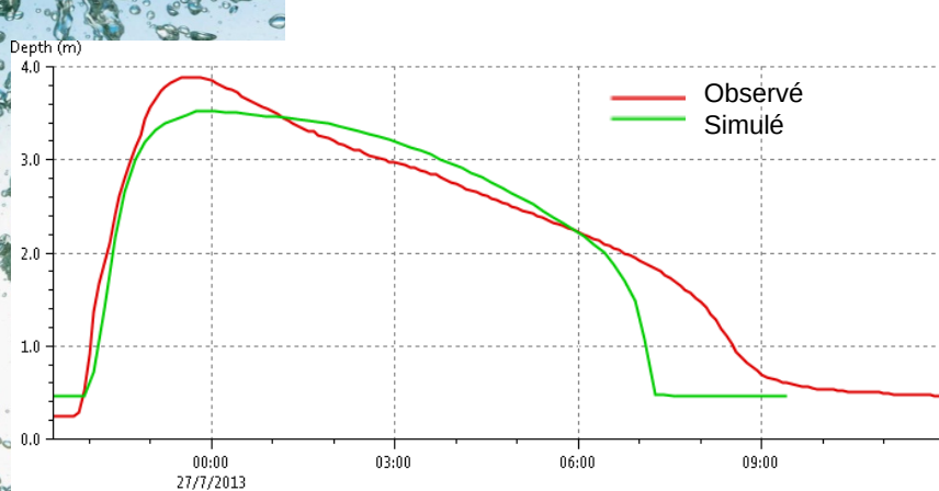
Exemple : Hauteur d'eau dans le bassin de Tresses
