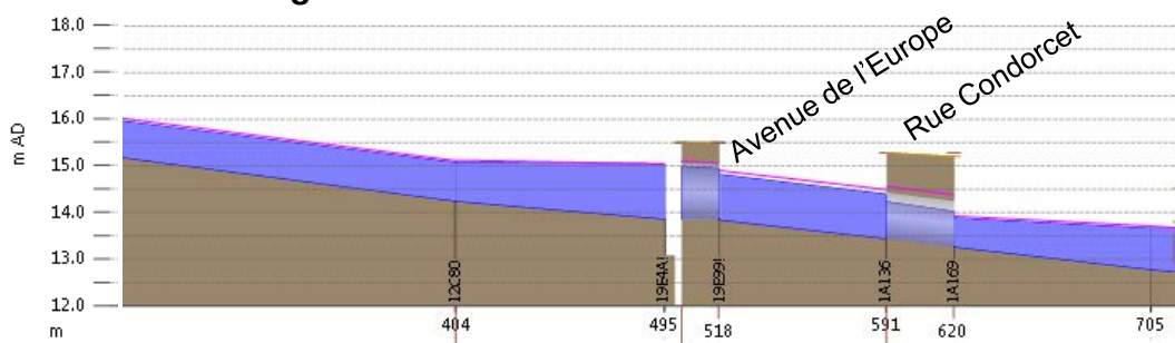
Profil en long – T = 20 ans
