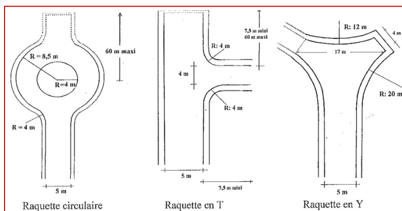
Aire de retournement pour voie en impasse d'une longueur supérieure à 60 mètres
