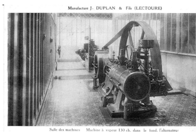
Fig. 6 - La machine à vapeur (Archives Municipales de Lectoure : carte postale 5Fi11).
