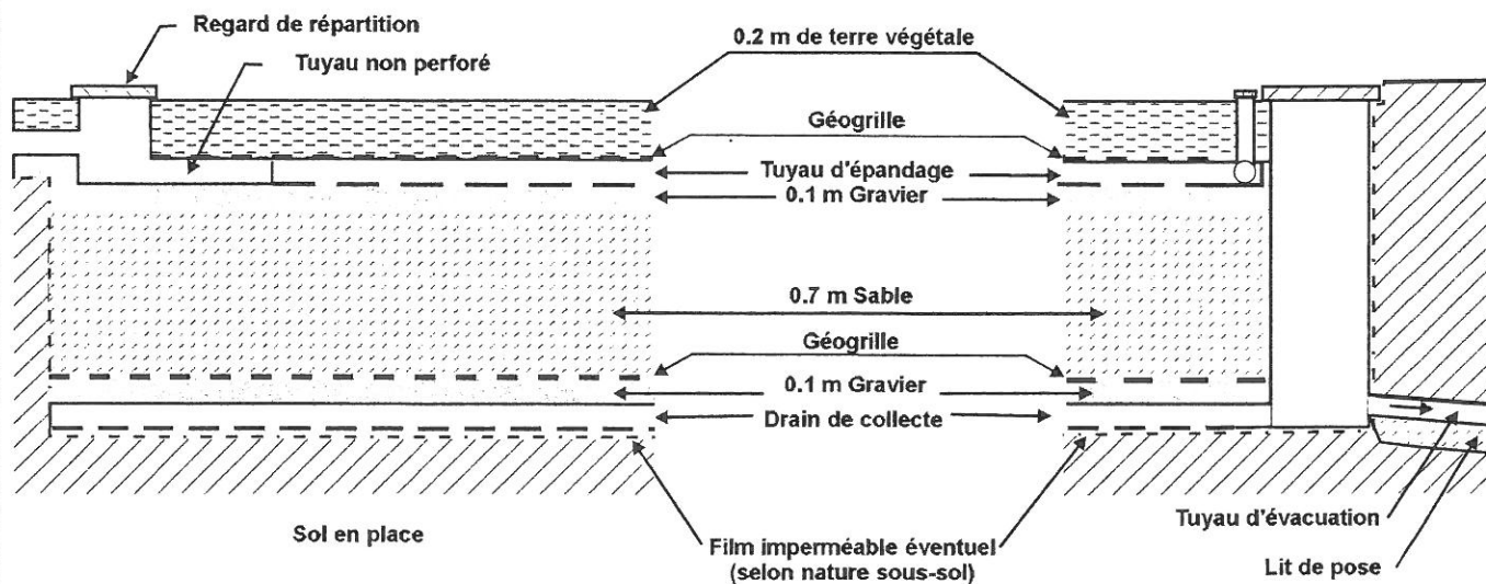
Coupe longitudinale
