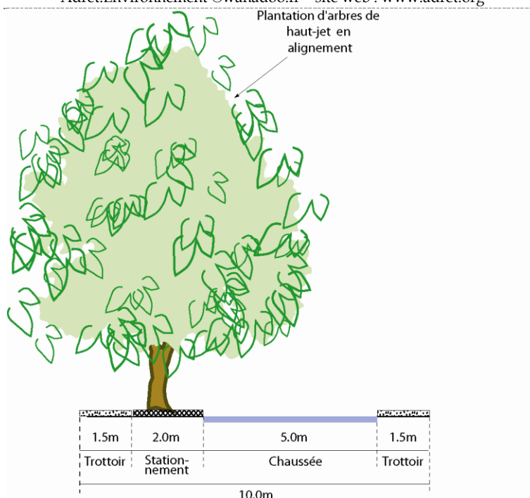
PROFIL-TYPE B DE LA VOIE PRIMAIRE (SANS LIAISON DOUCE)
