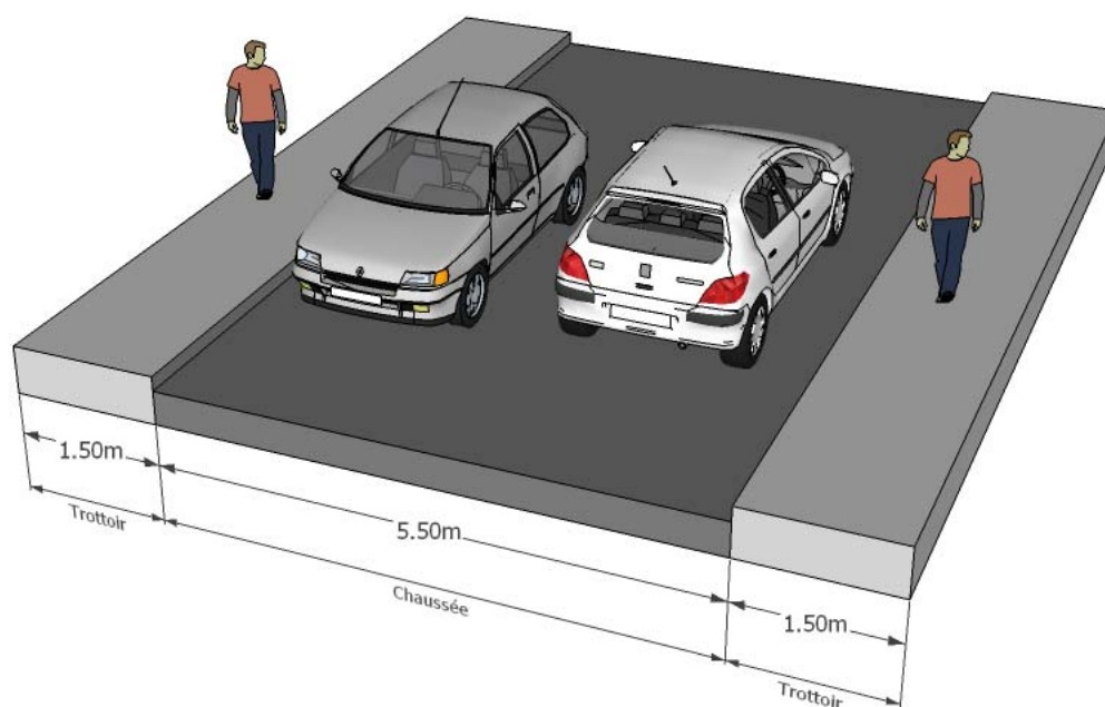
Coupe 1 : Proposition de principe d'aménagement d'une voie pour un lotissement d'habitation
