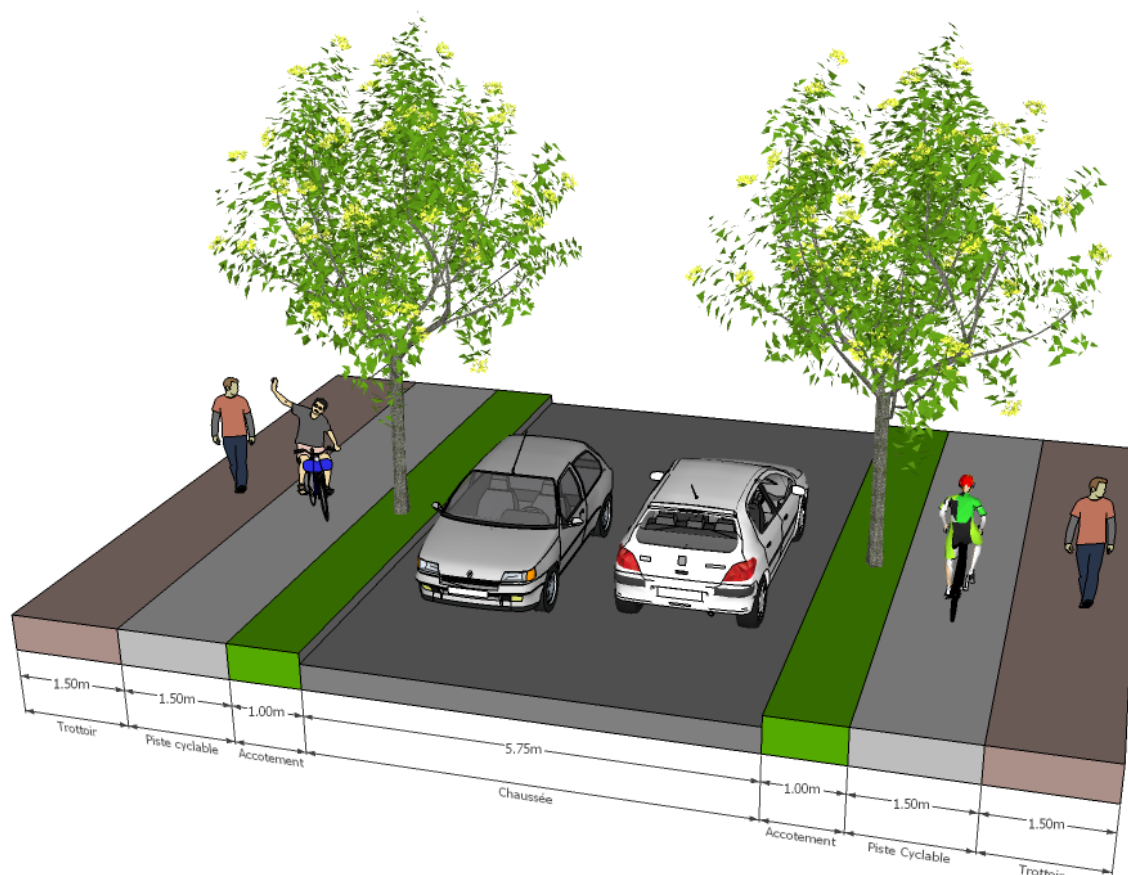
Coupe 2 : Proposition de principe d'aménagement d'une voie et de cheminements doux pour un lotissement d'habitation
