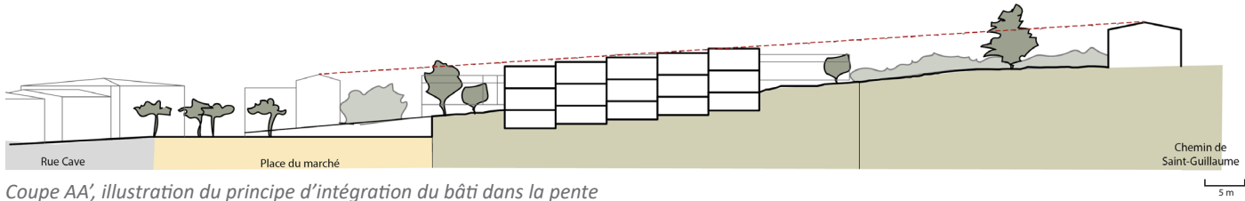
Coupe AA', illustration du principe d'intégration du bâti dans la pente
