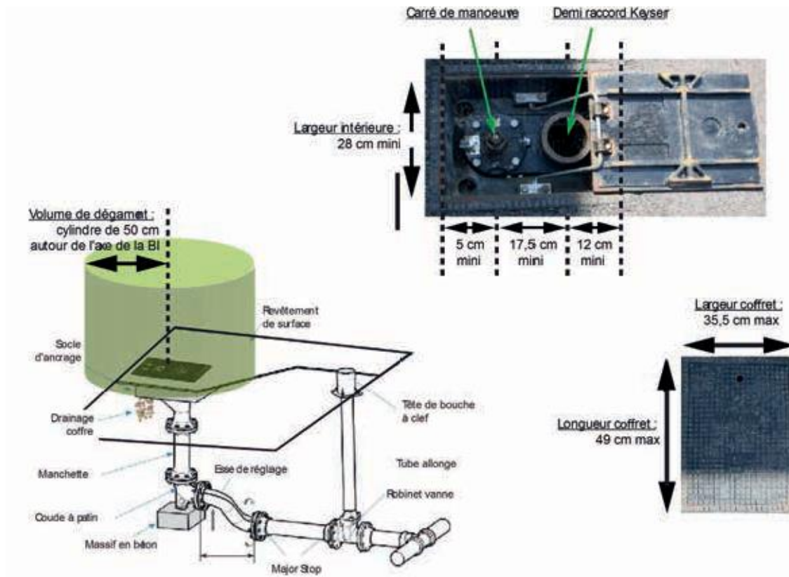
Figure 20 : Schéma d'implantation d'une BI normalisée
