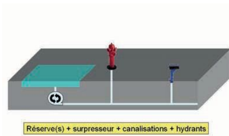
Figure 22 : Exemple n°2 d'une solution de réseau d'eau non potable
