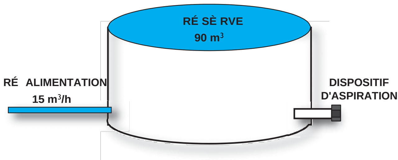
Figure 29 : Principe de réalimentation
