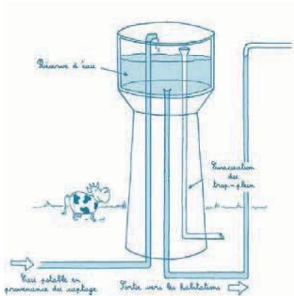
Figure 18 : Schéma de principe d'un château d'eau
