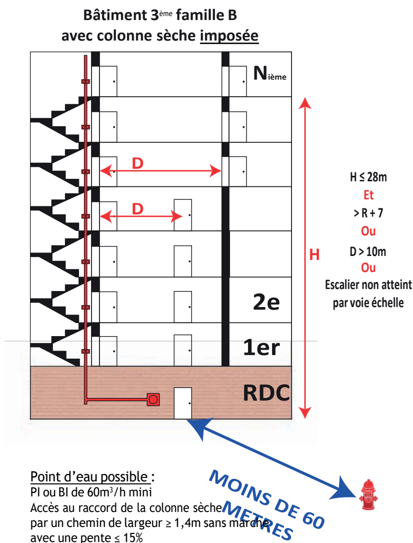
Figure 6 : Schéma de principe pour la couverture d'une habitation 3 ème famille B avec colonne imposée
