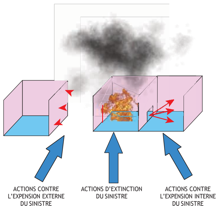
Figure 1 : actions d'extinction et de protection
