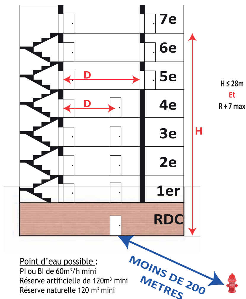
Figure 4 : schéma de principe pour la couverture d'une habitation 3 ème famille A ou B sans colonne sèche
