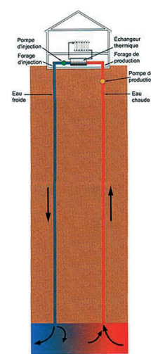
Principe du doublet géothermique
