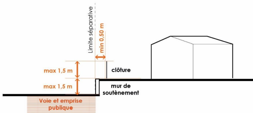
Schémas illustrant la règle
