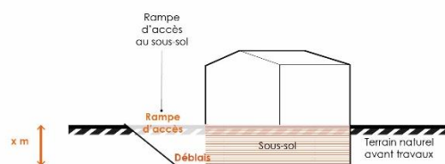
Schémas illustrant la règle
