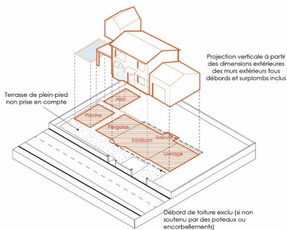
Emprise au sol
