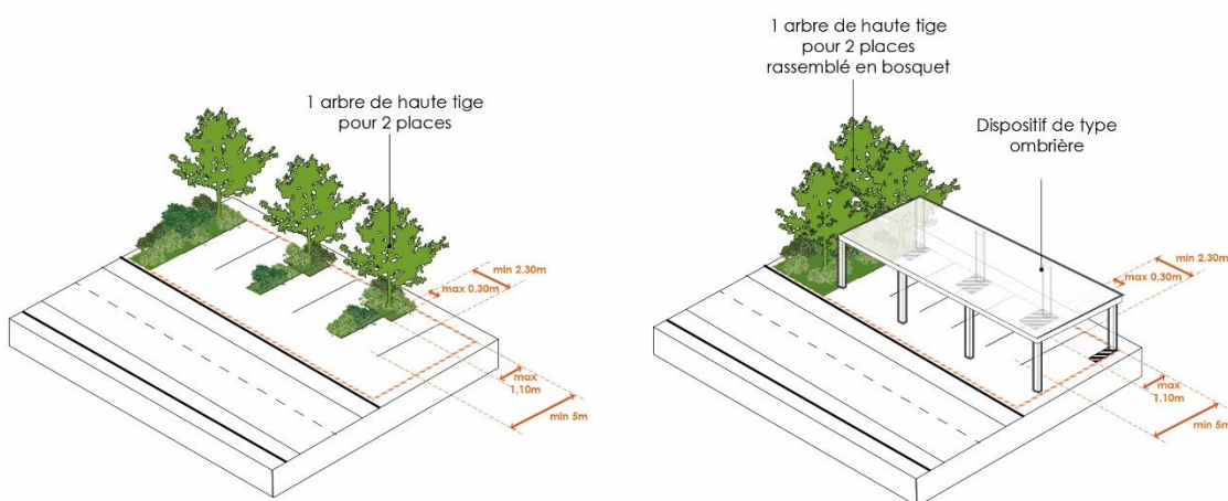
Schémas illustrant la règle
