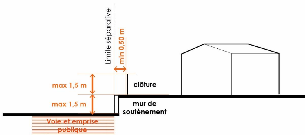
Schémas illustrant la règle
