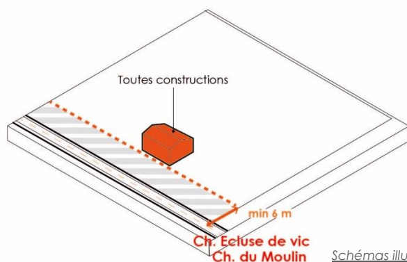
Schémas illustrant la règle
