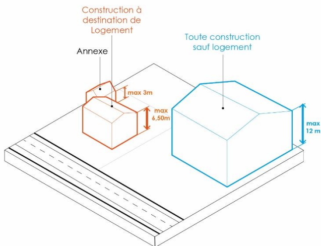
Schémas illustrant la règle
