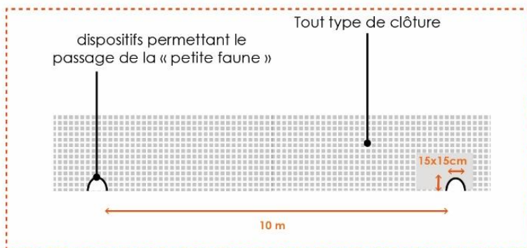
Schémas illustrant la règle
