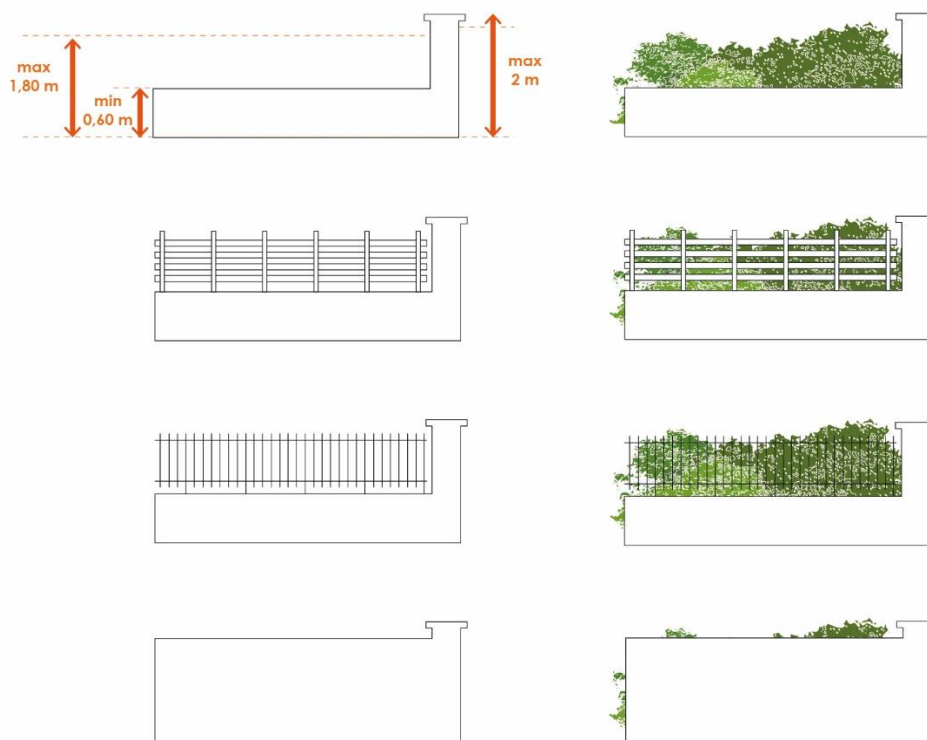
Schémas illustrant la règle
