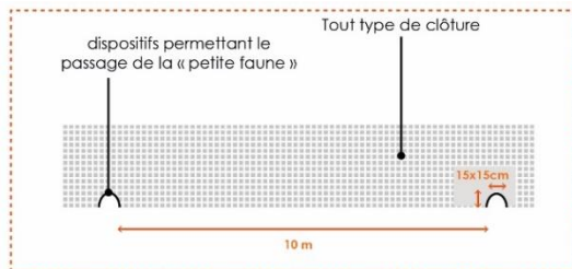
Schémas illustrant la règle
