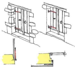
Transformation d'une ancienne porte d'étable en volet abattant sur la façade avec pose de pentures coudées.
