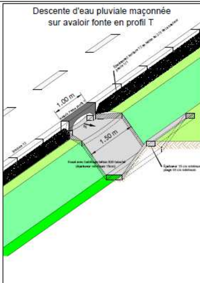
Descente d'eau pluviale maçonnée (épaisseur minimum 15cm)
