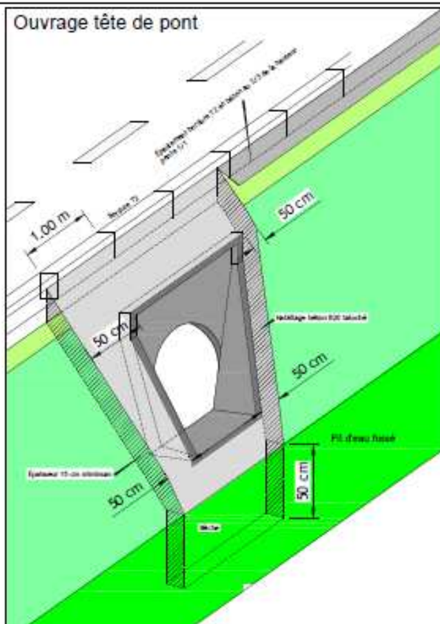
Tête d'aqueduc de sécurité
