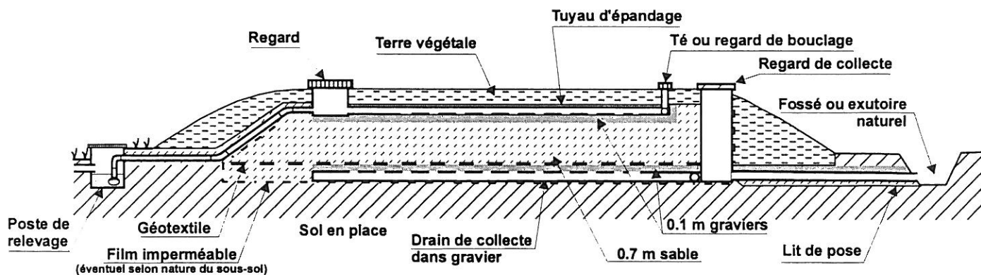
Coupe longitudinale
