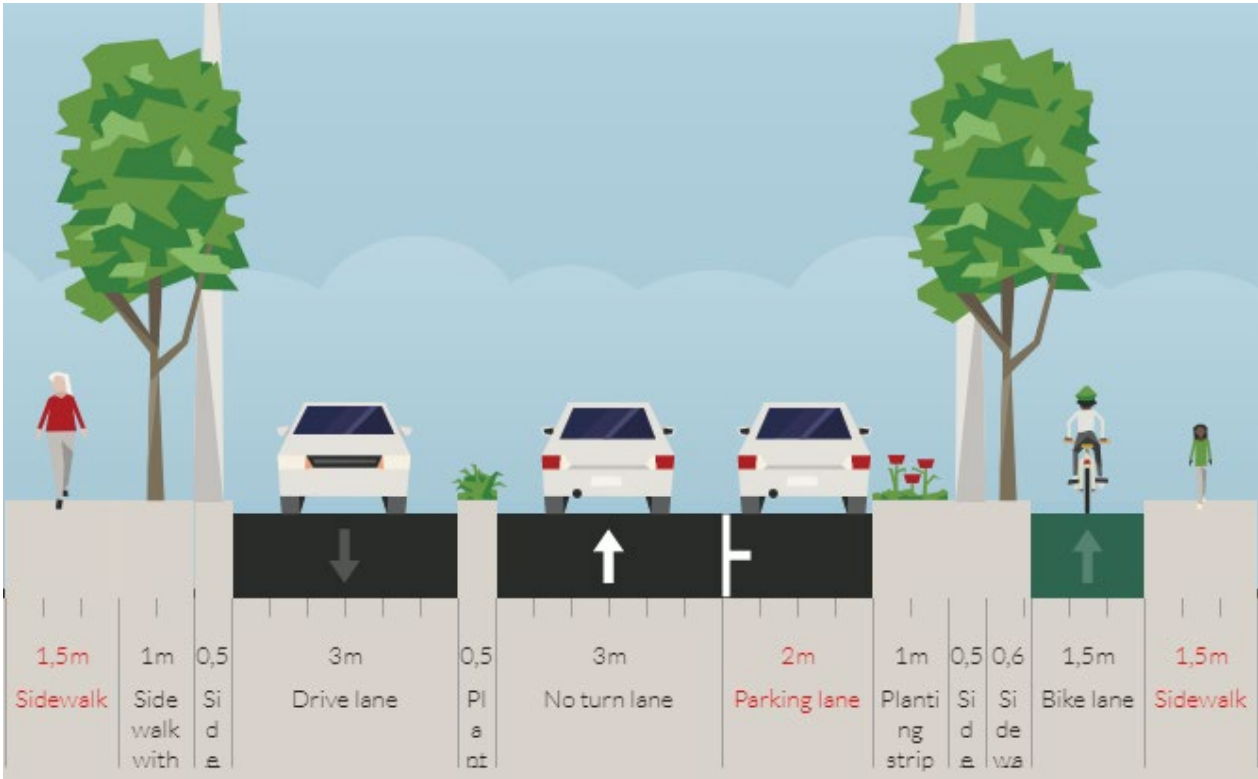
Exemple de profil de voirie principale à double-sens
