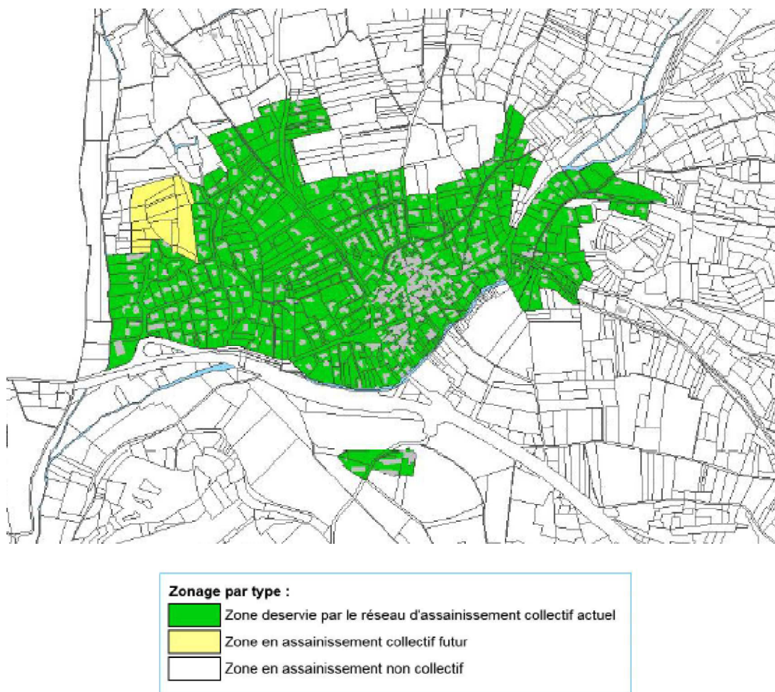
Extrait du zonage d'assainissement, OTEIS mars 2018
