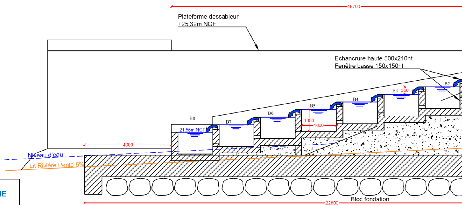
Coupe A4-A4 Passe à poissons
