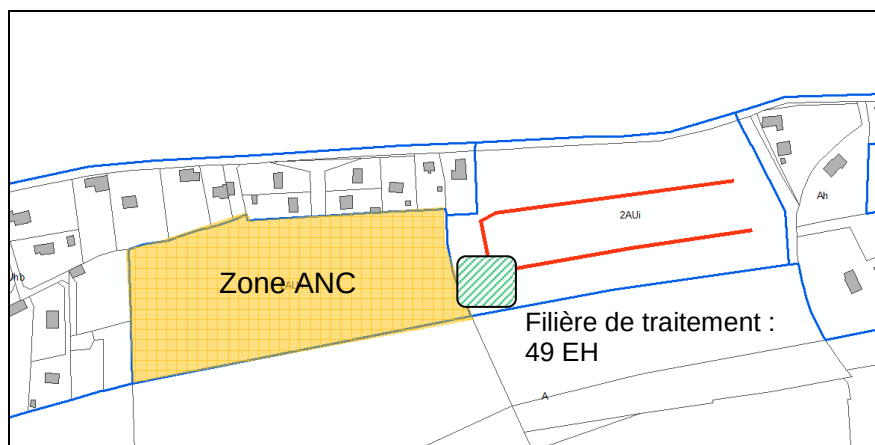
Figure 10 : Tracé schématique du réseau – scénario 2
