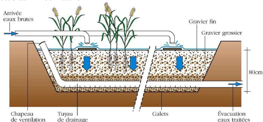
Figure 7 : Coupe transversale d'un filtre planté à écoulement vertical (source CEMAGREF)
