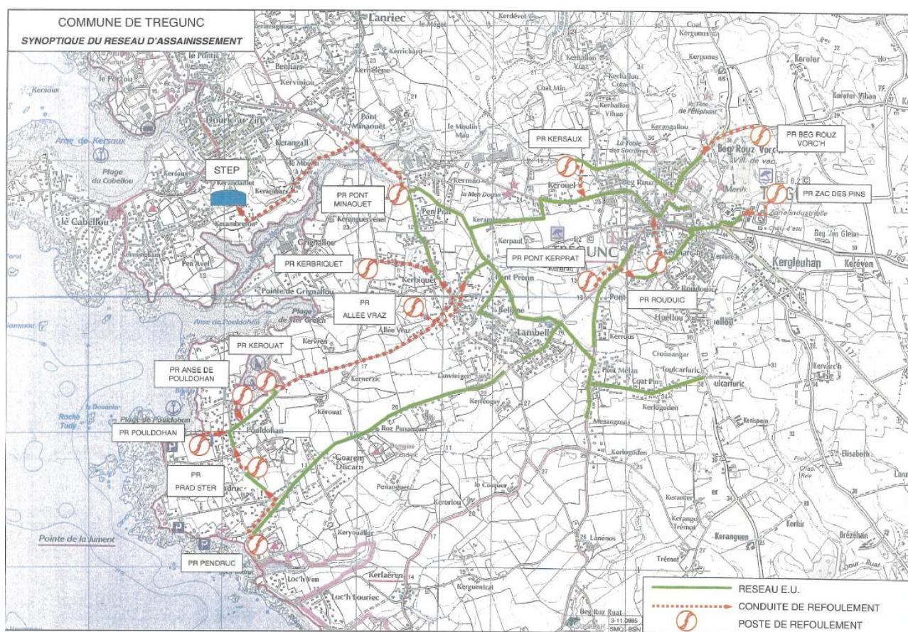
Figure 6 : Plan issu de l'étude diagnostique du réseau d'assainissement (SOGREAH-2006)
