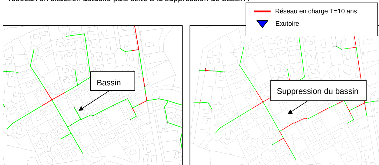
Figure 42 : Modélisation de la suppression du bassin de Kervinouel
