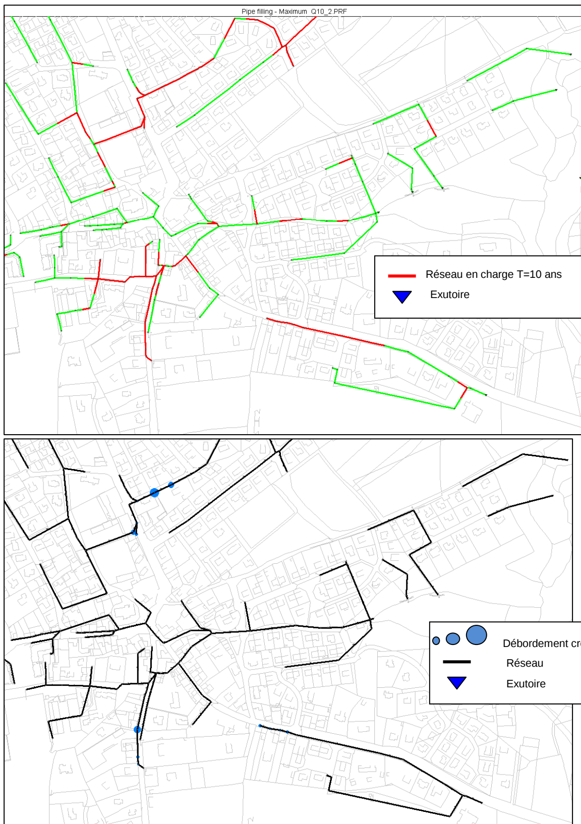
Figure 51 : Bassin versant de Lavoisier – Résultats en situation actuelle
