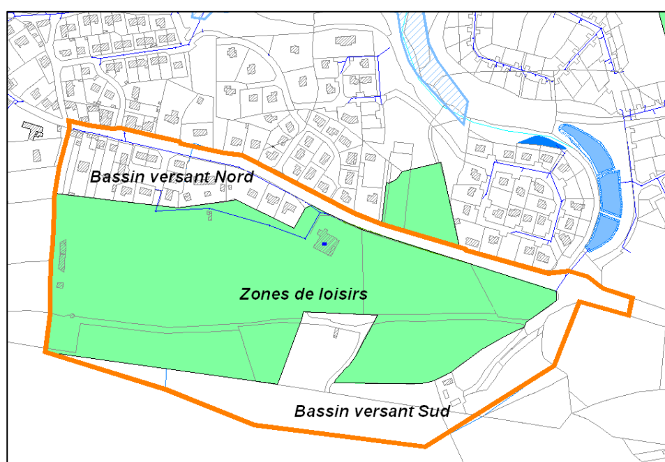
Figure 63 : Décomposition du bassin versant amont réel des bassins de Kergreiz
