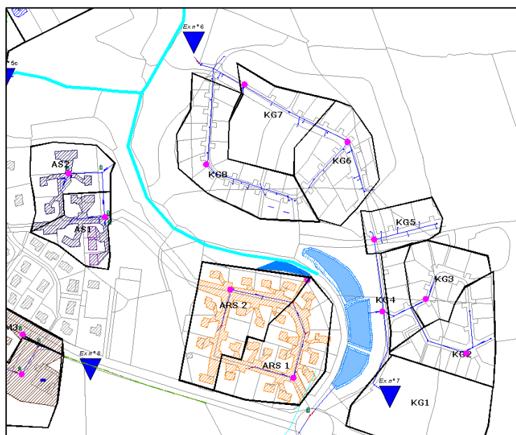
Figure 58 : Bassin versant de Kergreiz
