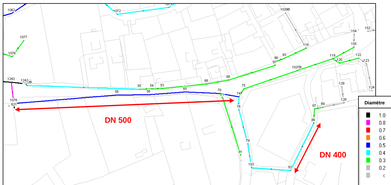
Figure 48 : Remplacement des réseaux Route de Pouldreuzic
