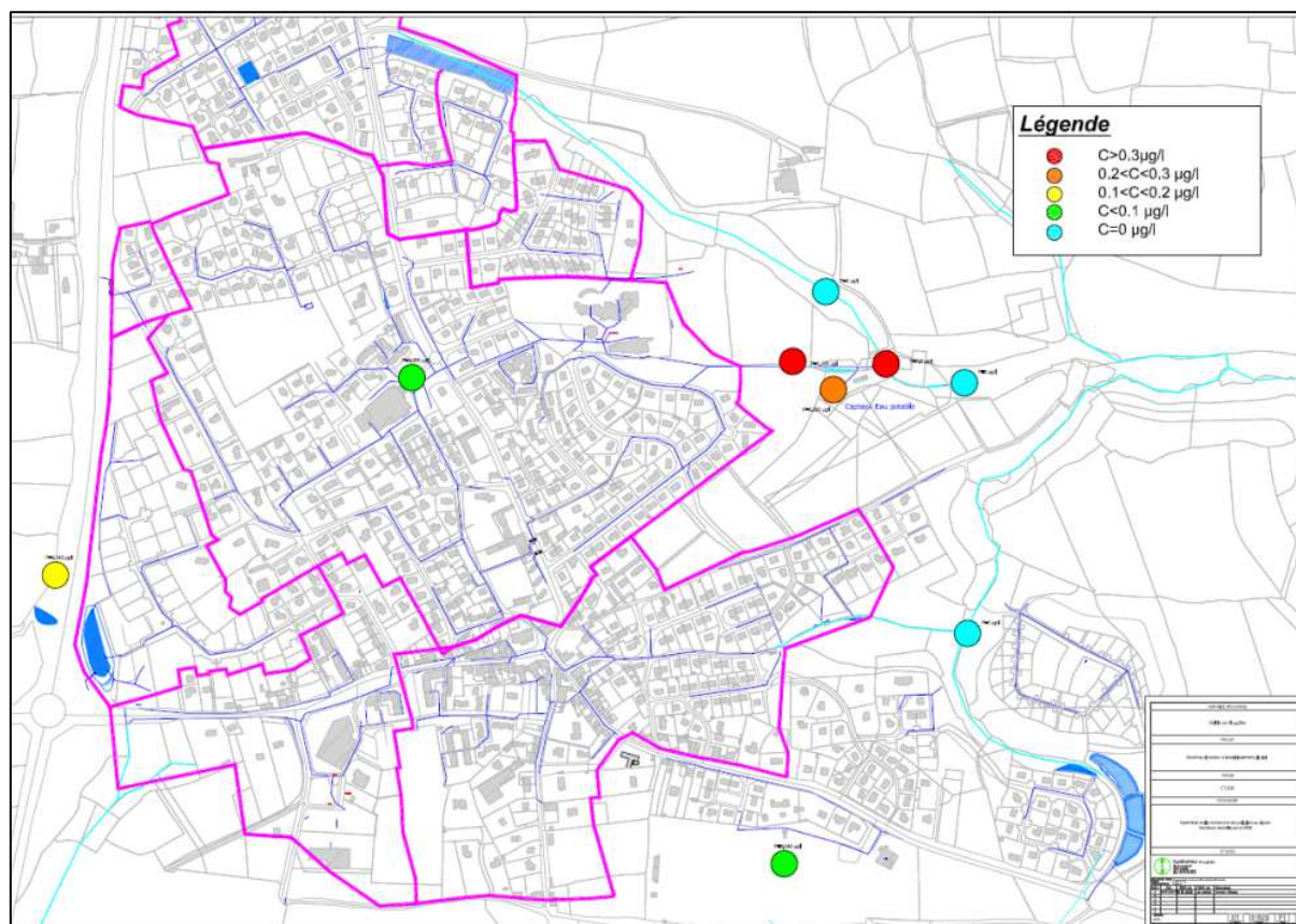
Figure 12 : Recherche de l'origine de la pollution
