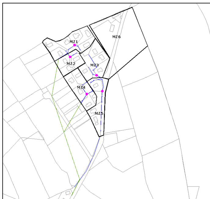
Figure 70 : Bassin versant de Menez Boutin
