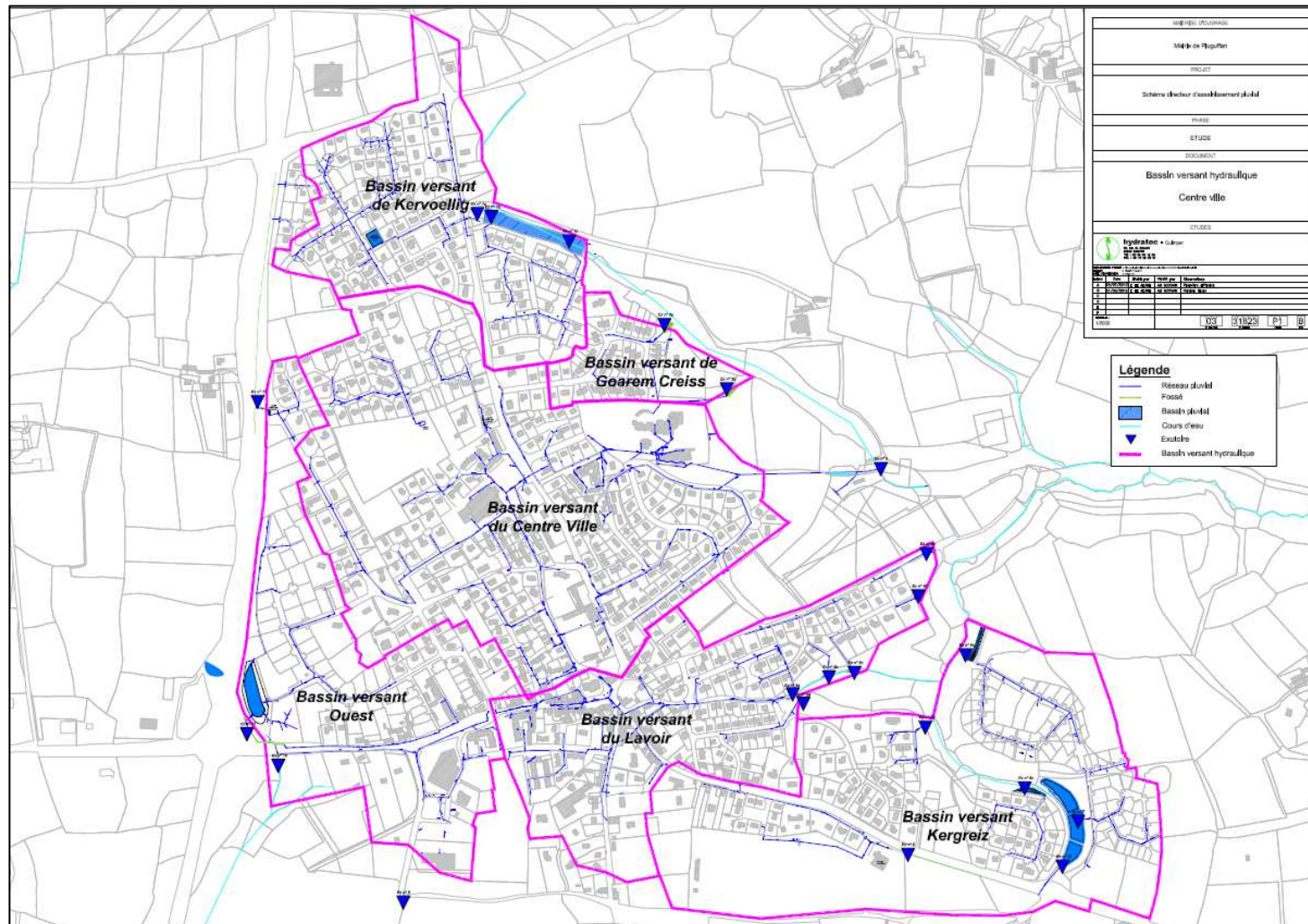
Figure 17 : Bassins versants sur la commune de Pluguffan
