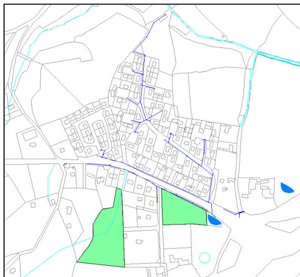
Figure 3 : Commune de Pluguffan – Urbanisation envisagée à Kermaduit et Treger Greiz
