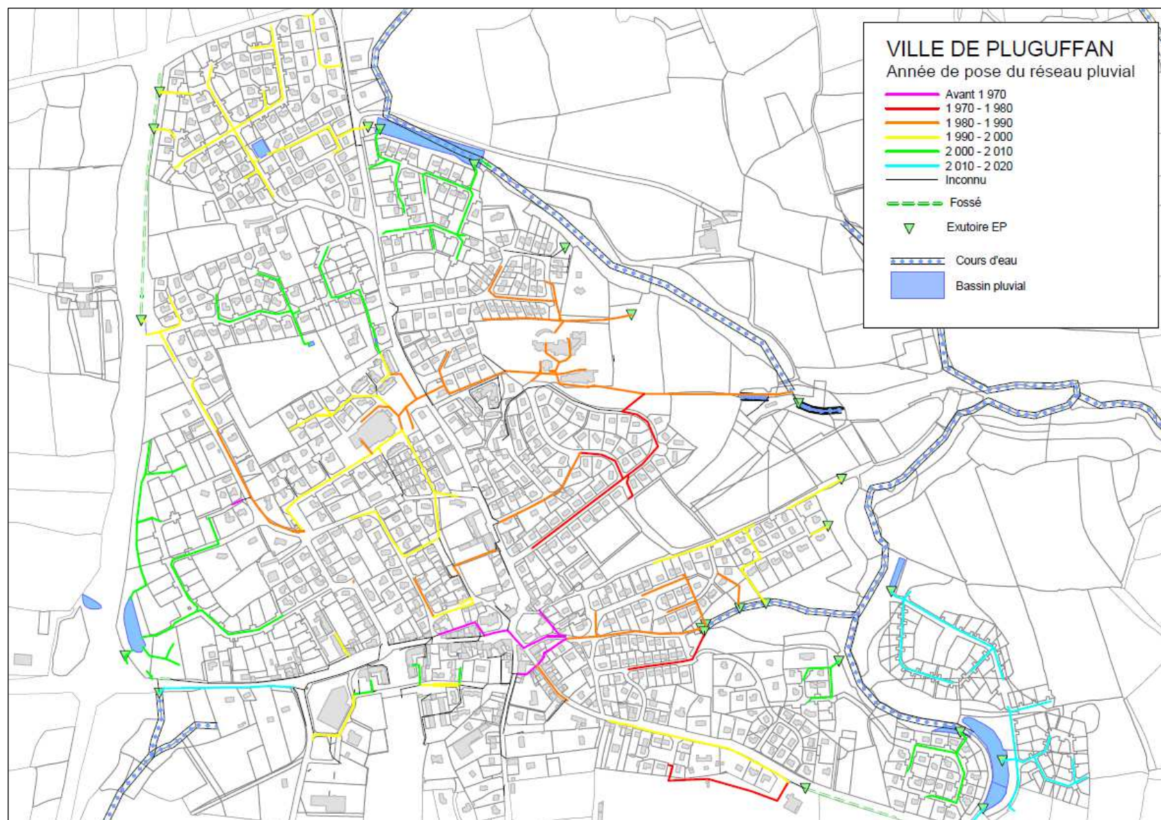
Figure 8 : Année de pose des réseaux
