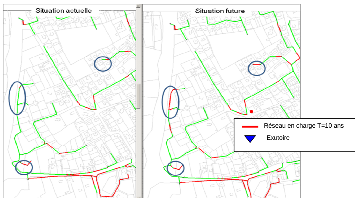
Figure 47 : Modélisation du bassin versant de Ty Pin en situation future
