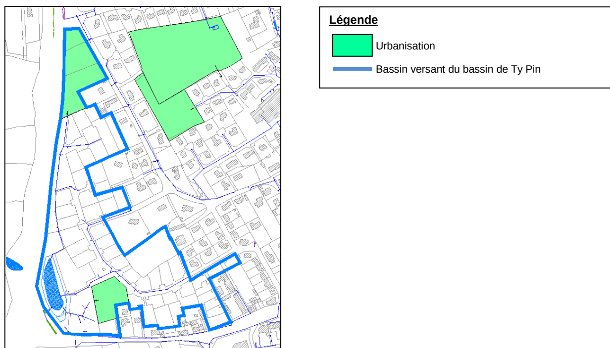
Figure 46 : Bassin versant du bassin de Ty Pin existant
