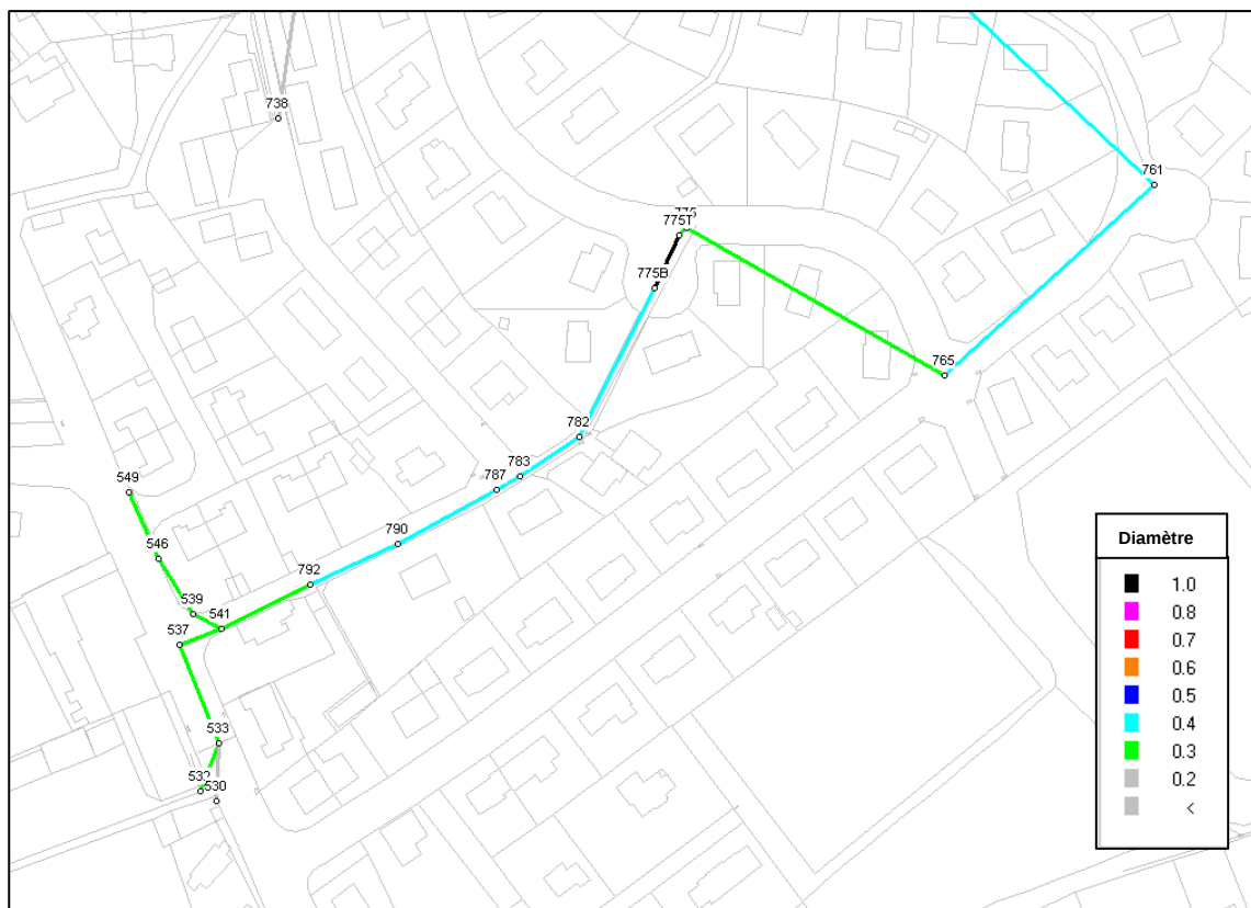
Figure 26 : Scénario 4 - Création d'une rétention enterrée
