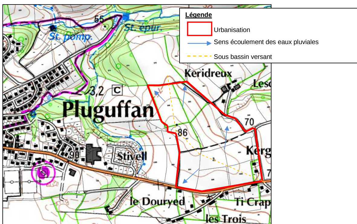
Figure 60 : Localisation de Kergreiz 3 et de ses sous bassins versants
