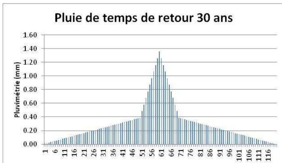
Figure 15 : Pluviogramme de la pluie de période de retour 30 ans
