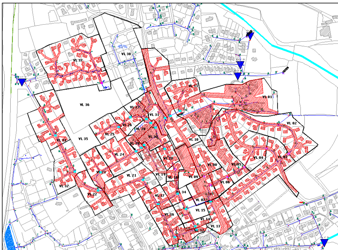
Figure 19 : Bassin versant du Centre Ville
