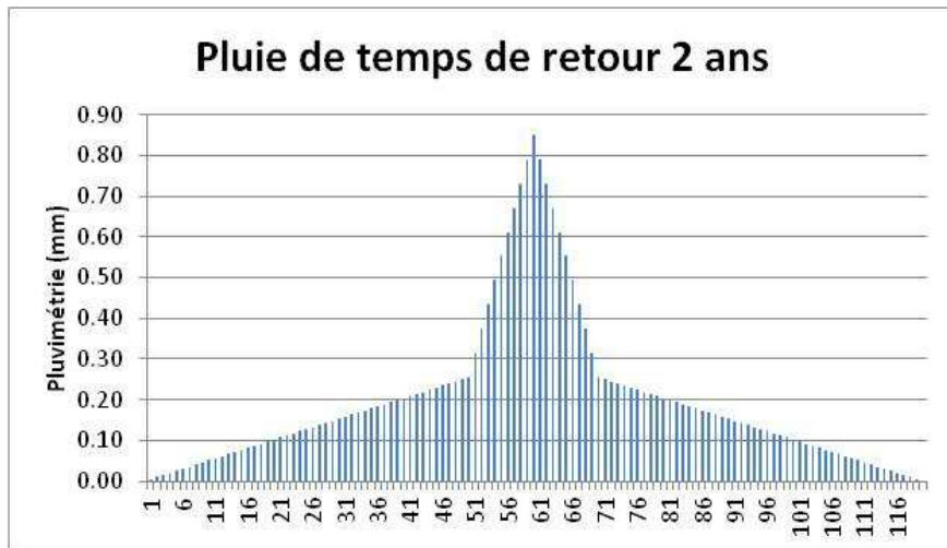
Figure 13 : Pluviogramme de la pluie de période de retour 2 ans
