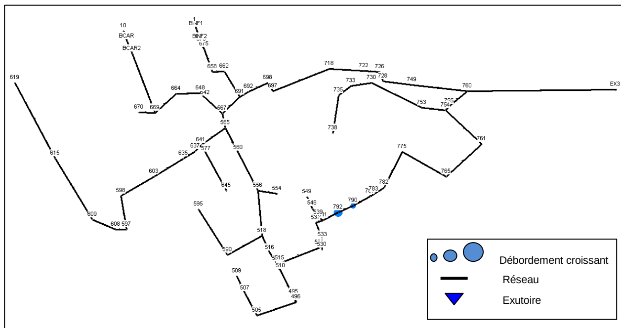
Figure 20 : Débordements au Centre Ville pour une pluie 2 ans
