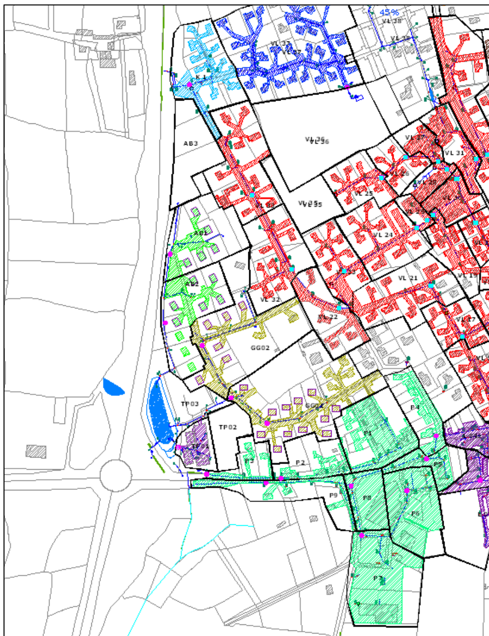
Figure 44 : Découpage en bassins versants du secteur Ouest
