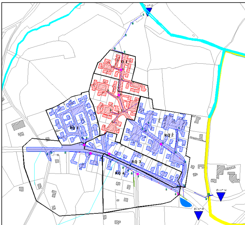
Figure 65 : Bassin versant du Treger Greiz
