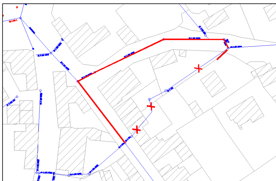
Figure 54 : Déviation des réseaux entre rue de Quimper et rue du Lavoir
