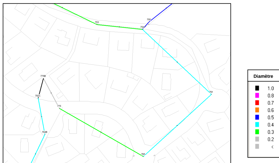
Figure 29 : Scénario 4b - Modélisation réalisée
