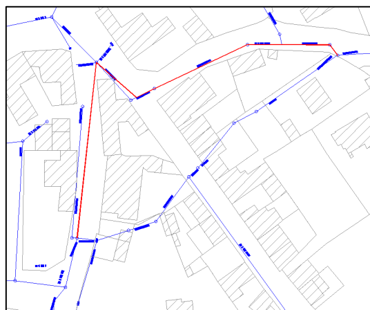
Figure 55 : Déviation des réseaux entre rue du Stade et rue du Lavoir
