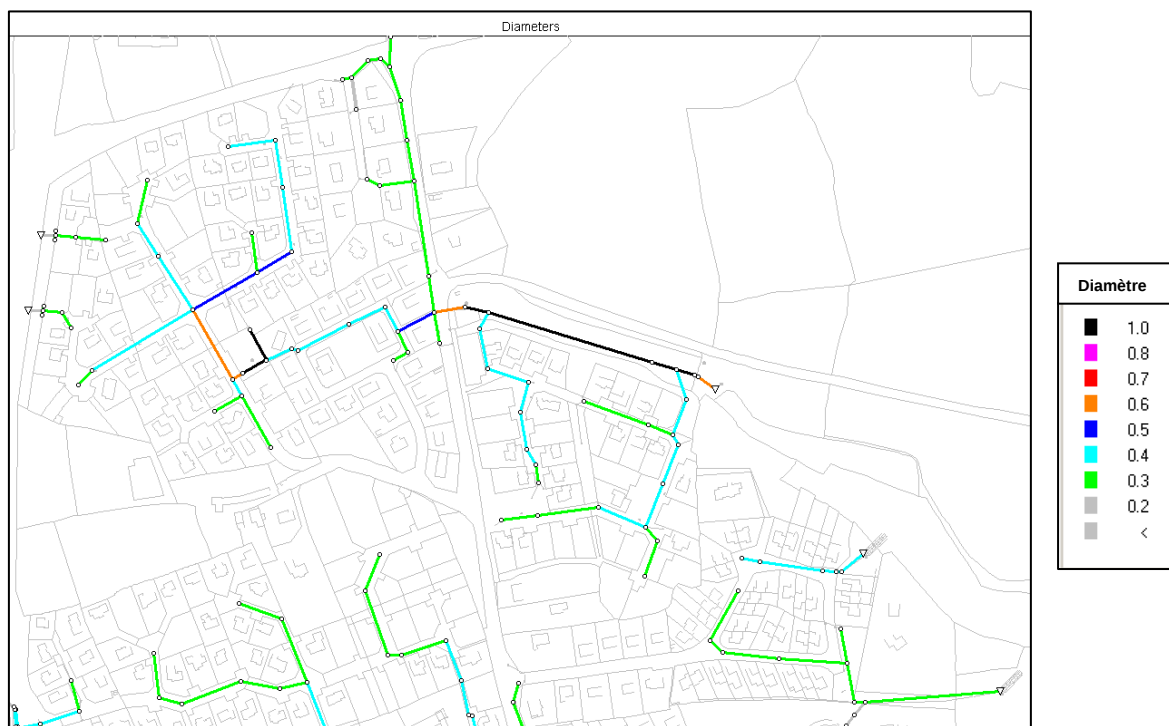
Figure 34 : Caractéristiques du réseau de Kervoellig
