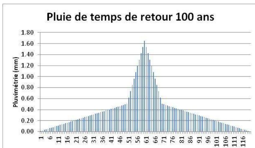
Figure 16 : Pluviogramme de la pluie de période de retour 100 ans
