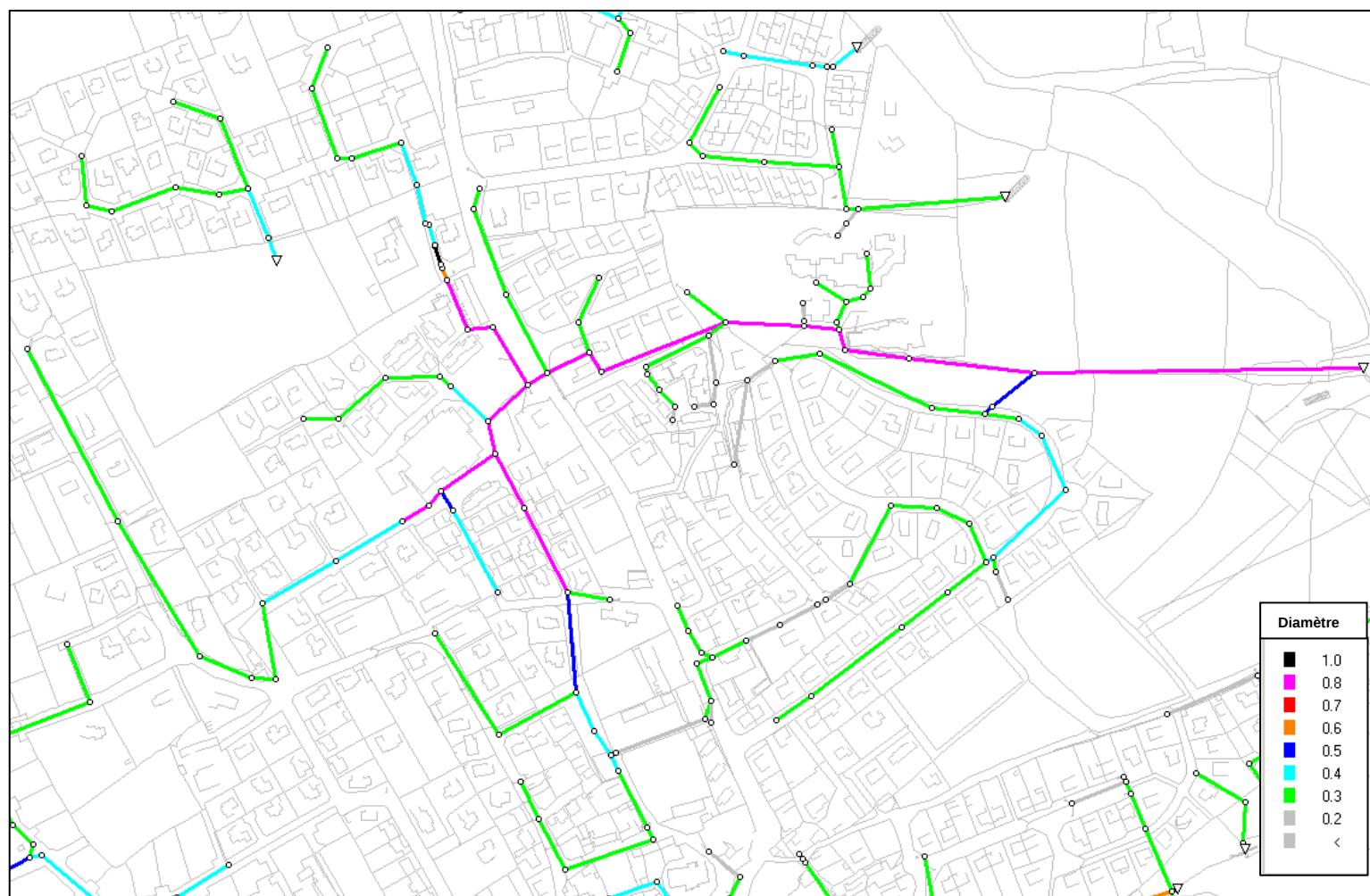
Figure 18 : Caractéristiques des réseaux - Bassin versant du Centre Ville
