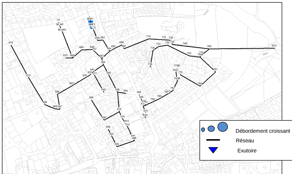
Figure 30 : Vérification du scénario 3 pour une pluie 30 ans
