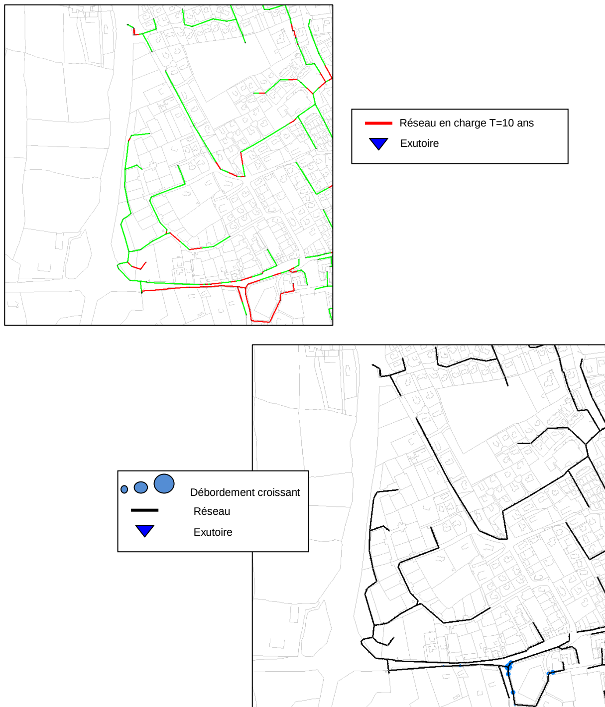
Figure 45: Bassin versant Ouest – Débordements Pluie 10 ans
