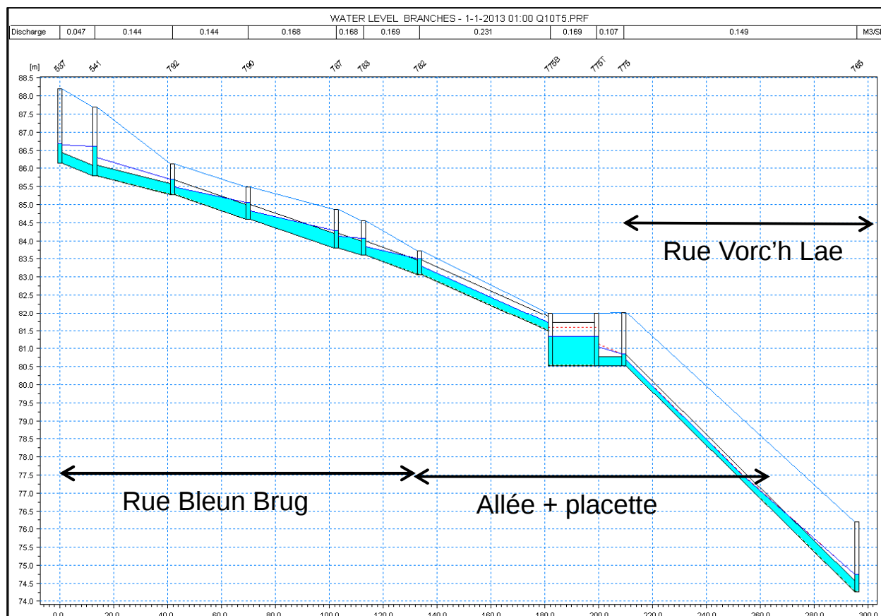
Figure 27 : Scénario4 - Profil en long avec bassin enterré
