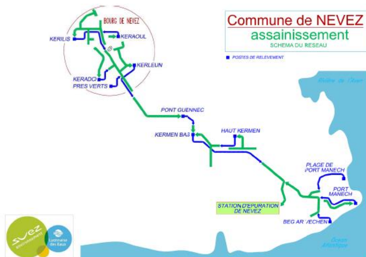
Schéma du réseau d'assainissement de la commune de Névez
