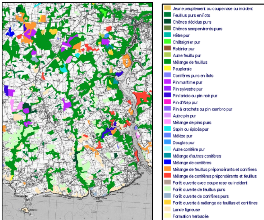
Typologie des boisements sur la commune de Névez
