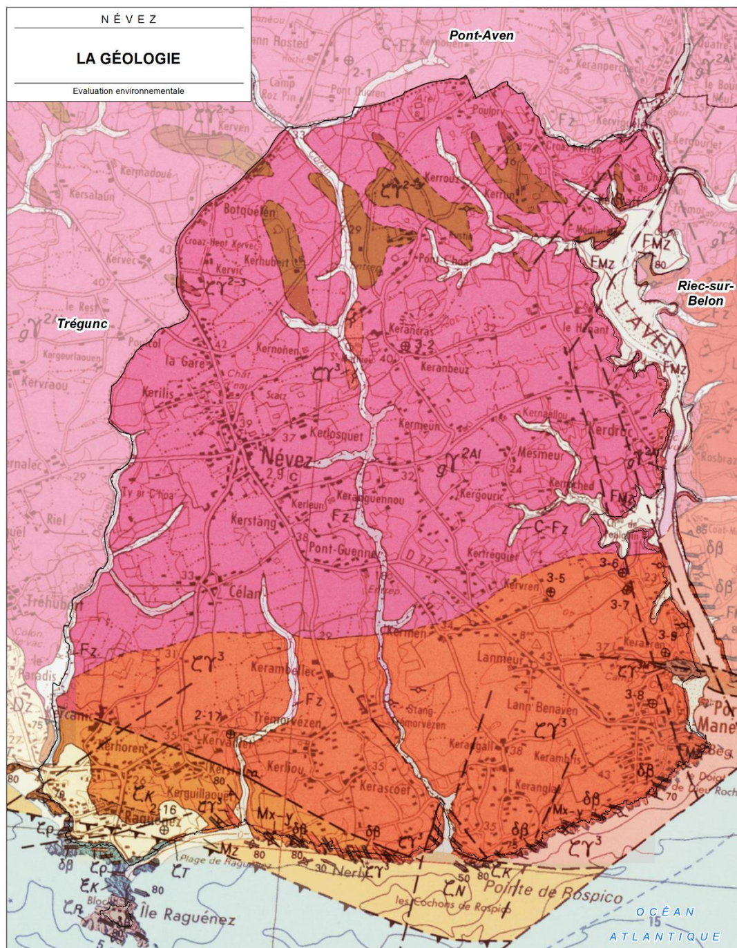
Légende de la carte géologique
