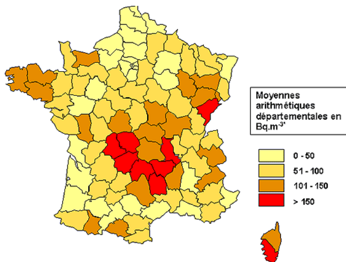
Activités volumiques du radon dans les habitations
