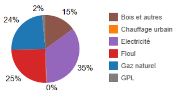
Répartition des résidences principales par énergie principale de chauffage à l'échelle de Concarneau Cornouaille Agglomération
