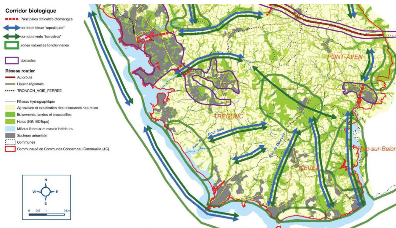
Fonctionnement écologique globale du territoire du SCoT de Concarneau Cornouaille Agglomération
