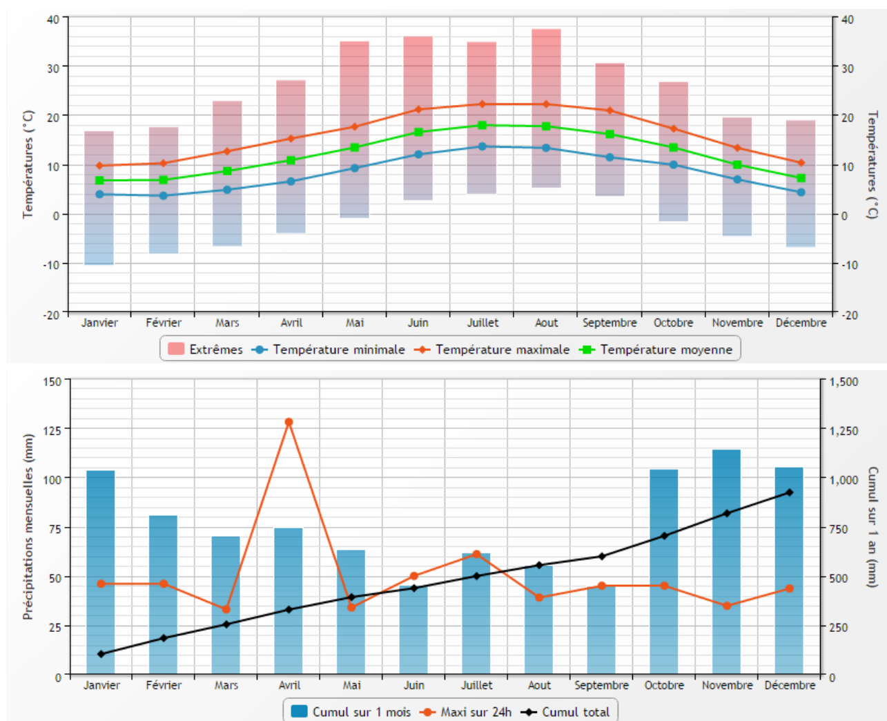
Températures (en haut) et précipitations (en bas) mensuelles à la station de Lorient-Lann Bihoué entre 2000 et 2015
