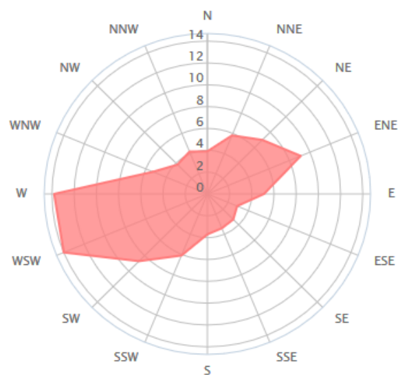
Rose des vents annuelle entre 11/2000 et 08/2016 à l'aéroport de Lorient Bretagne Sud
