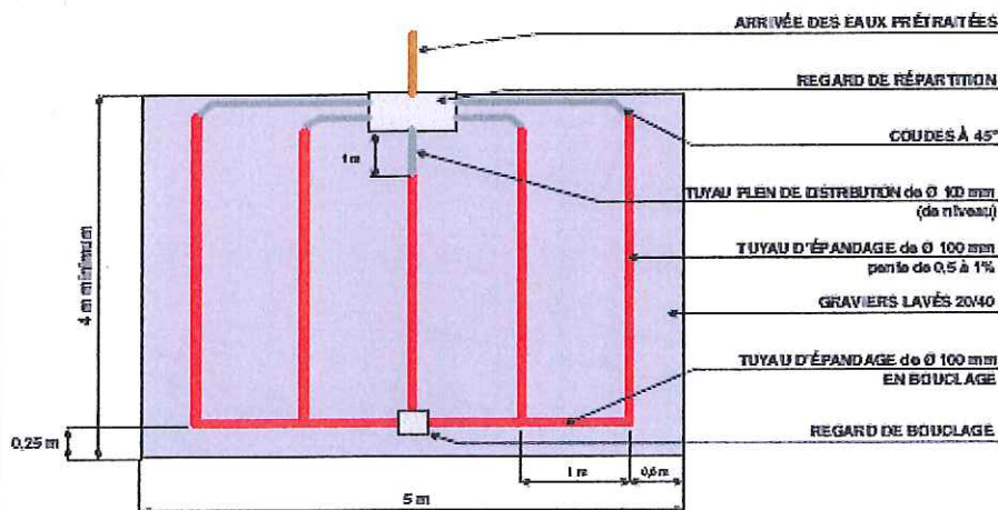
VUE DU DESSUS
