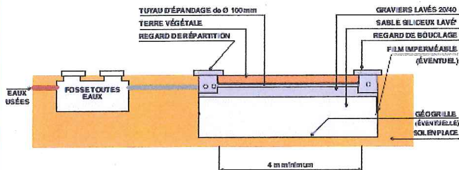
COUPE LONGITUDINALE
