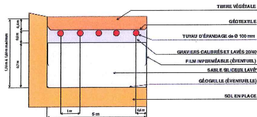
COUPE TRANSVERSALE
