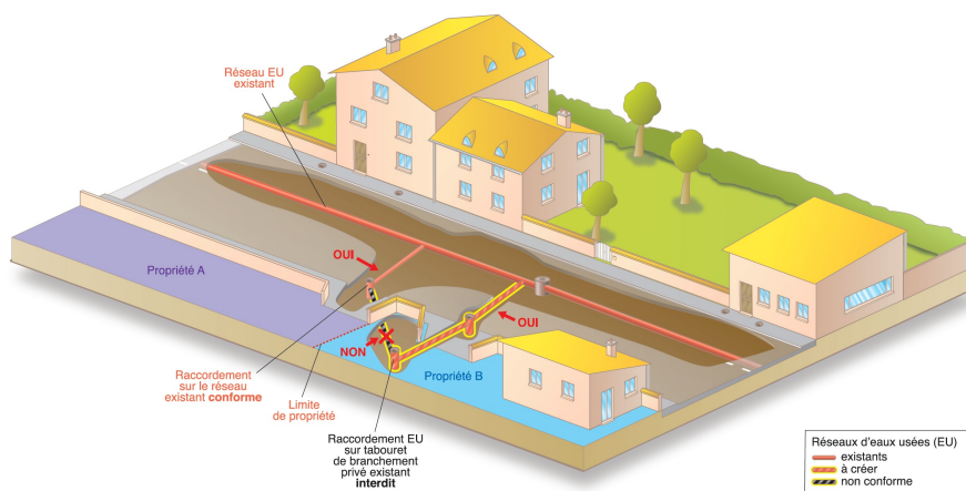
Fig 9 : raccordement interdit
