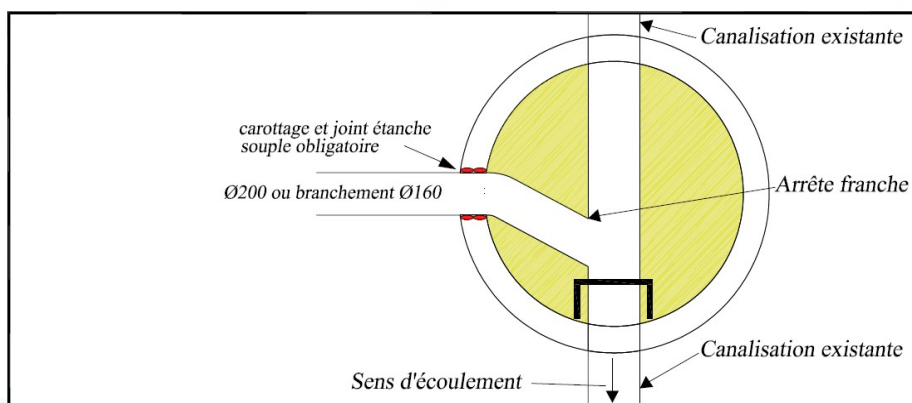
Fig 17 : raccordement sur banquettes, cas de h < 0,50\text{m} , vue de haut
