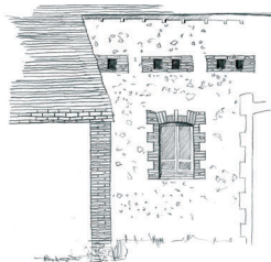
Maçonnerie mixte, enduit et brique : - tuiles plates en terre cuite, - chaîne d'angle et encadrements de baie en brique, - enduit à pierre vue en arrière plan, - enduit couvrant au premier plan.
