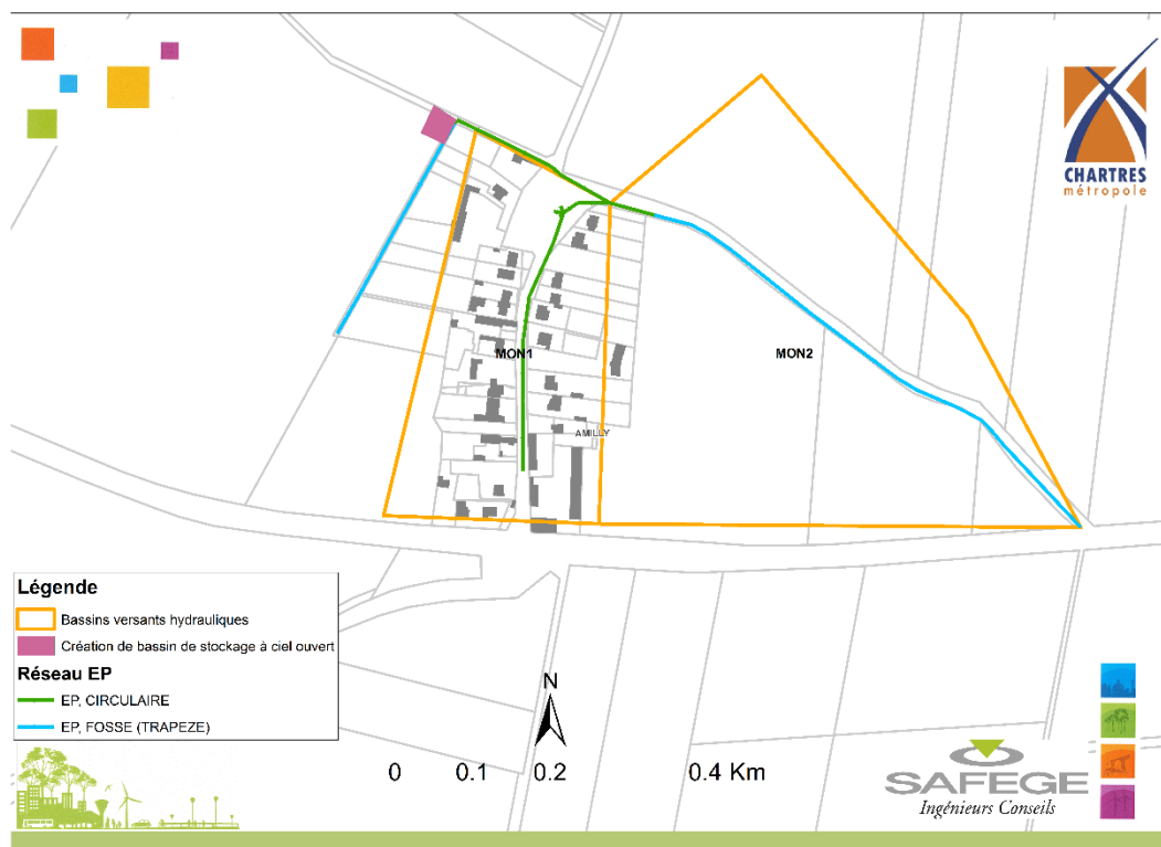
Figure 3-6 : Schéma de principe de la solution hydraulique proposée à Amilly
