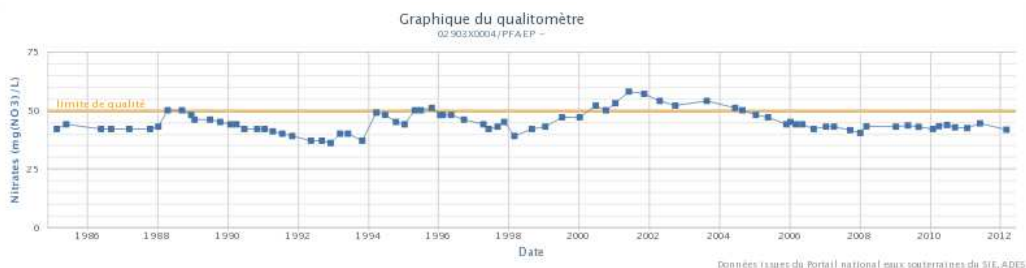
Figure 4-47 : Evolution des teneurs en nitrates dans le forage de Mérobert entre 1985 et 2013
