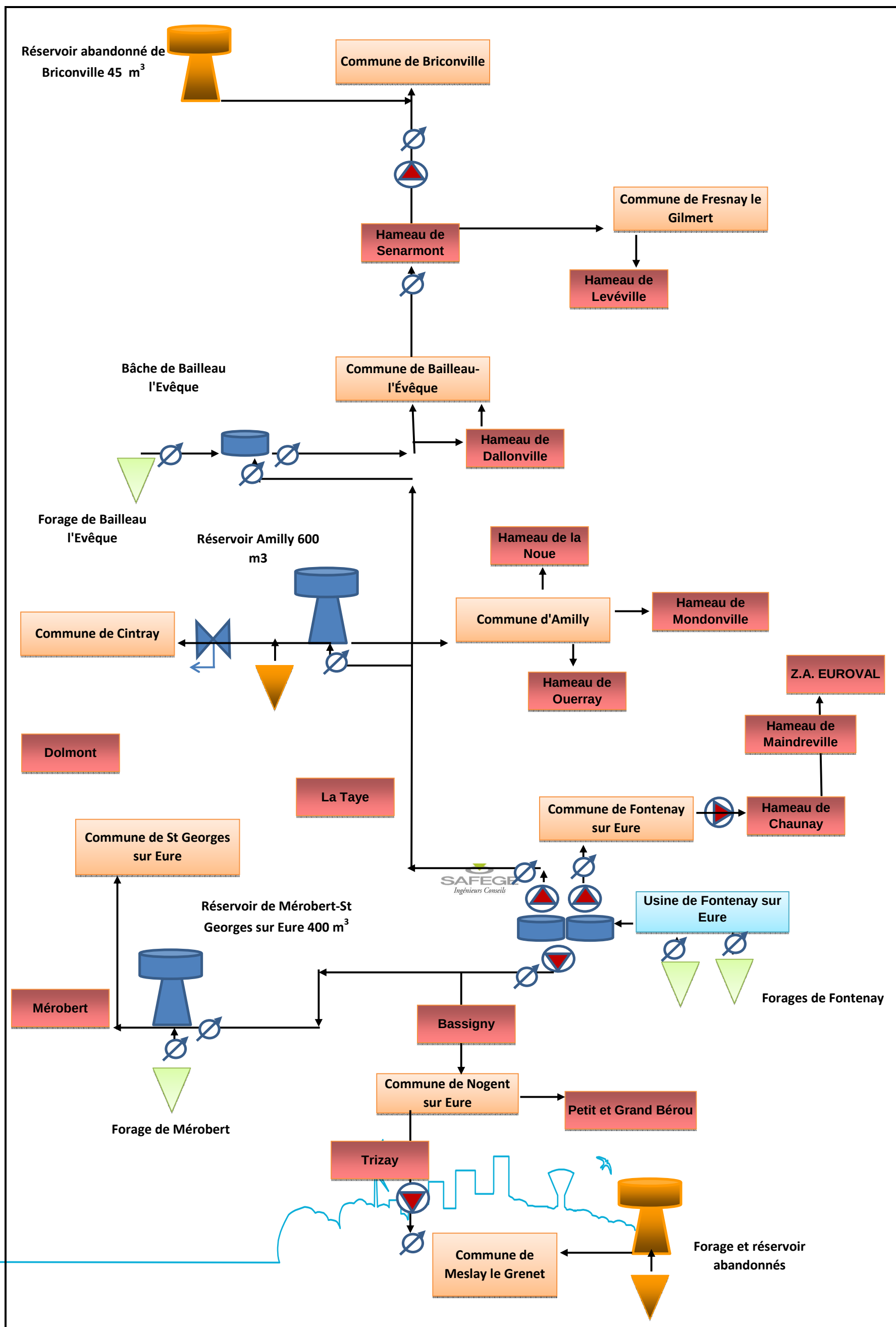
Figure 4-45 : Synoptique de fonctionnement du système de Fontenay-Amilly-Bailleau L'Évêque-St Georges
