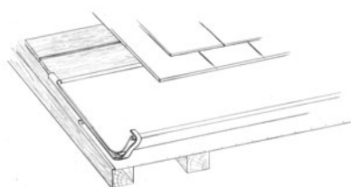
C - Gouttière havraise (ou nantaise) posée sur l'égout de toit.
