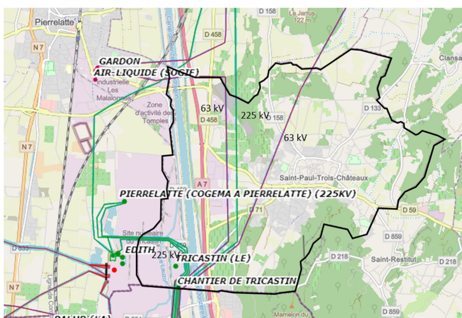
Réseau électrique sur la commune : Source : RTE
