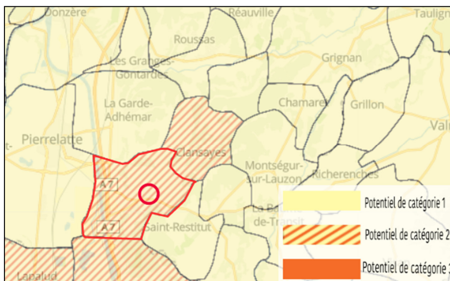
Potentiel radon de Saint-Paul-Trois-Châteaux (Source : IRSN)
