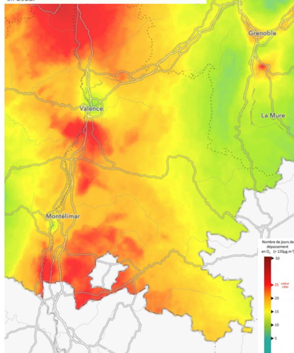
Nombre de jours "pollués" à l'ozone O 3 dans l'air ambiant, estimée par modélisation sur la région Auvergne-Rhône-Alpes, en 2022.
