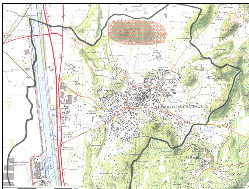
Cartographie de risque minier dans l'emprise de la commune
