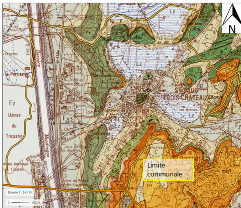
Extrait de la carte géologique au 1/50 000ème (N°890 – Valréas, BRGM)
