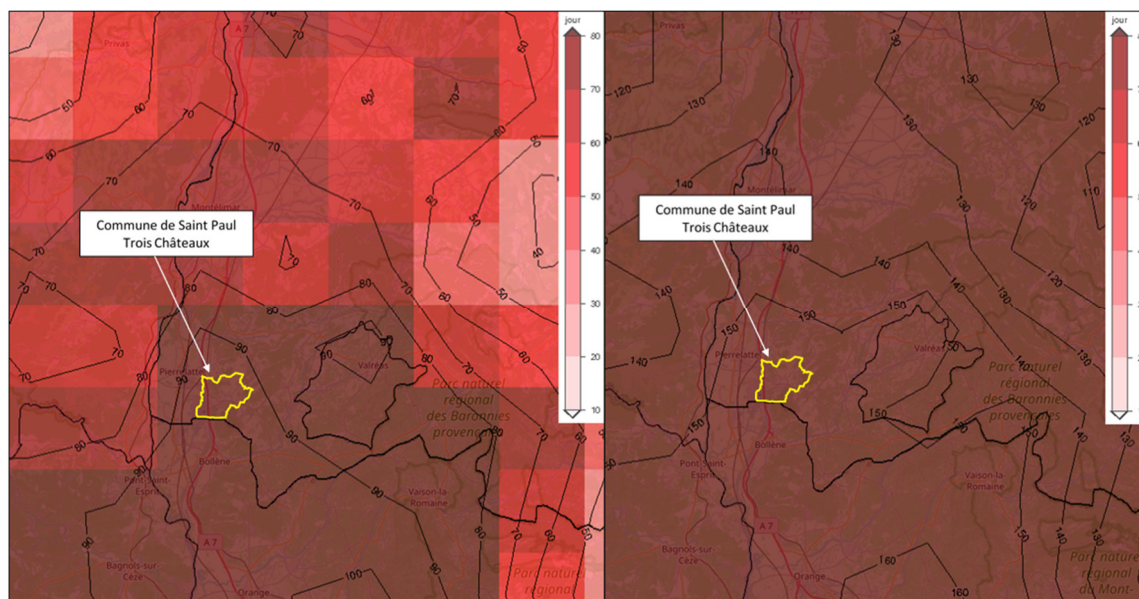
Modélisation des journées chaudes sur la commune de Saint Paul 3 Châteaux en état actuel (à gauche) et à l'horizon 2071-2100 (à droite) (Source : Drias)
