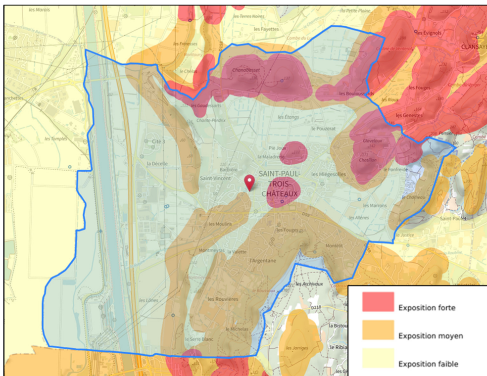
Extrait du site Géorisque et de l'Aléa retrait/gonflement des argiles centré sur la commune.
