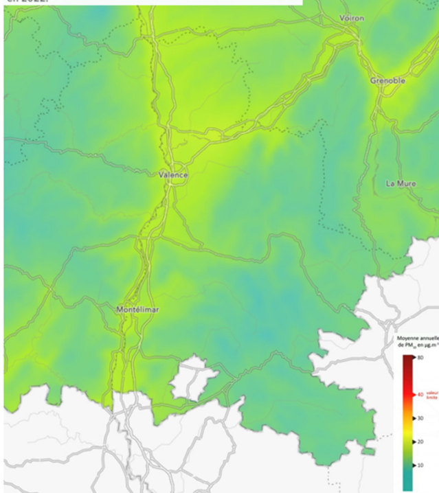
Moyenne annuelle de particules PM 10 dans l'air ambiant, estimée par modélisation sur la région Auvergne-Rhône-Alpes, en 2022.
