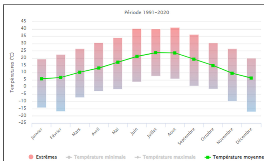
Températures sur la station météorologique de Montélimar-Ancone entre 1991 et 2020 (Source : Infoclimat)
