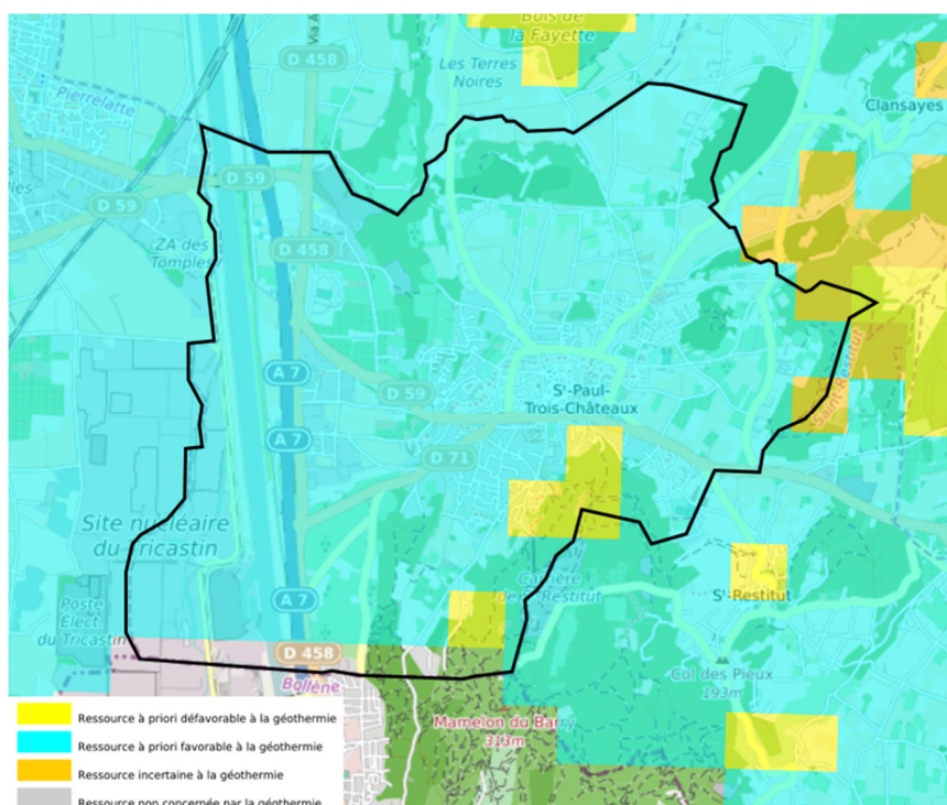
Ressource géothermique du sous-sol – Source : Géothermies.fr
