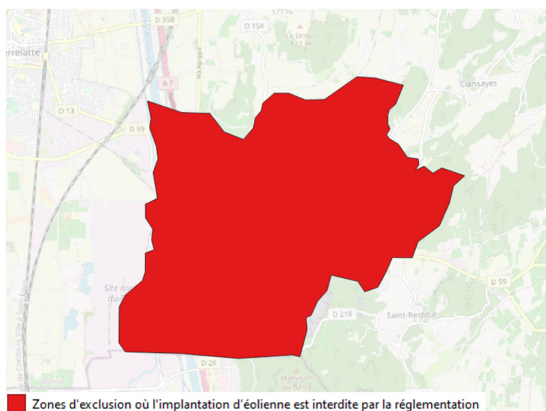
Potentiel éolien sur le territoire communal – Source : Schéma éolien 2019
