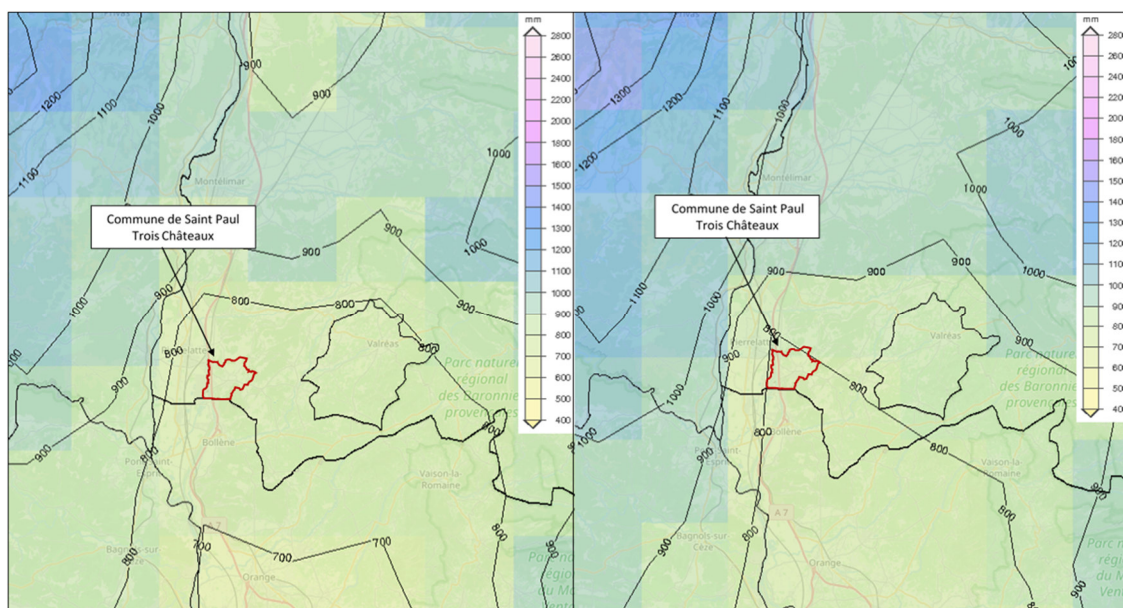
Modélisation des cumuls de précipitations sur la commune de Saint-Paul-3 Châteaux en état actuel (à gauche) et à l'horizon 2071-2100 (à droite) (Source : Drias)
