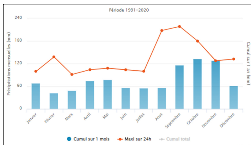
Cumuls pluviométriques mensuels de la station météorologique de Montélimar-Ancone entre 1991 et 2020 (Source : Infoclimat)
