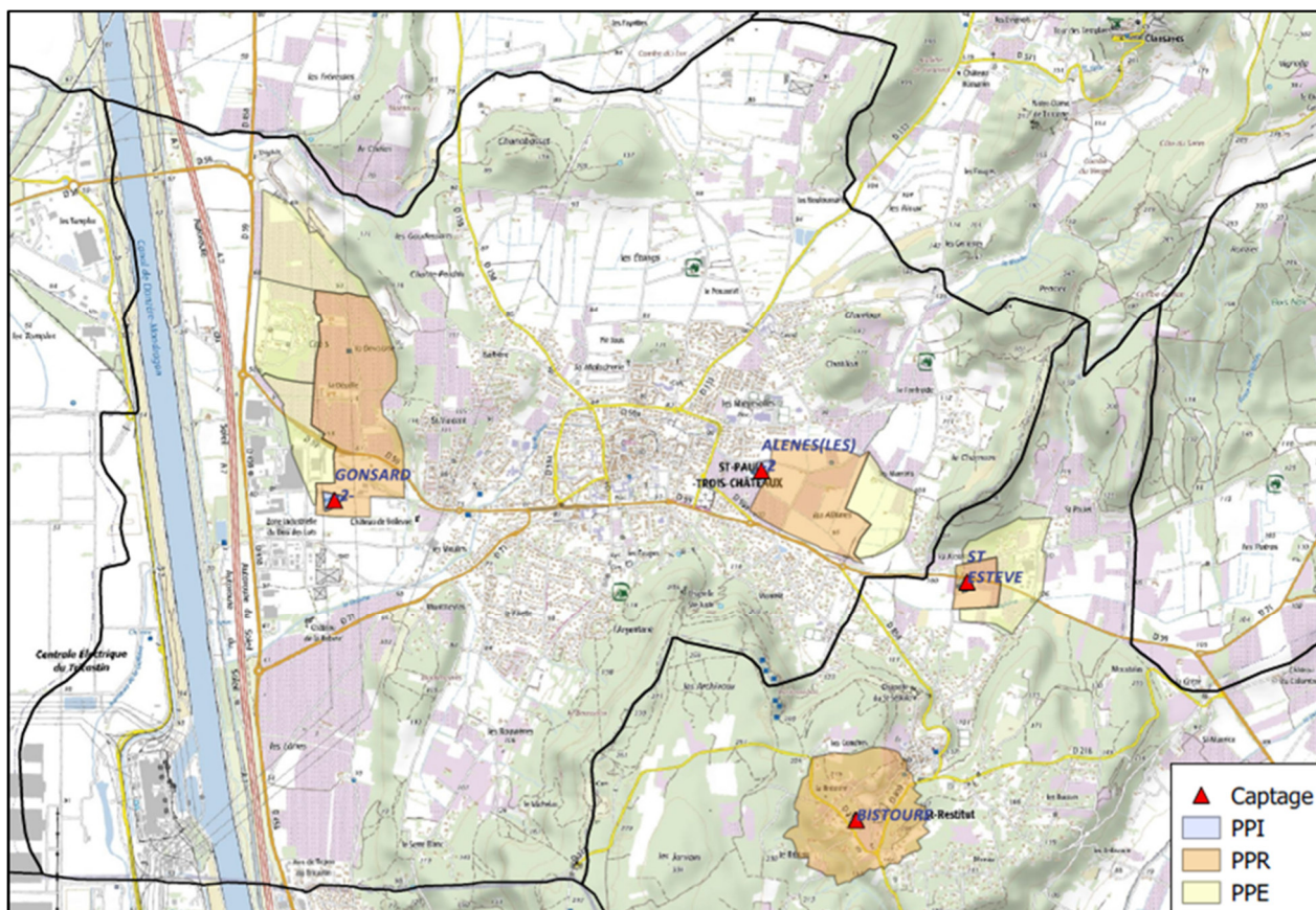
Localisation des captages AEP et de leurs périmètres de protection à Saint-Paul-Trois-Châteaux - ARS
