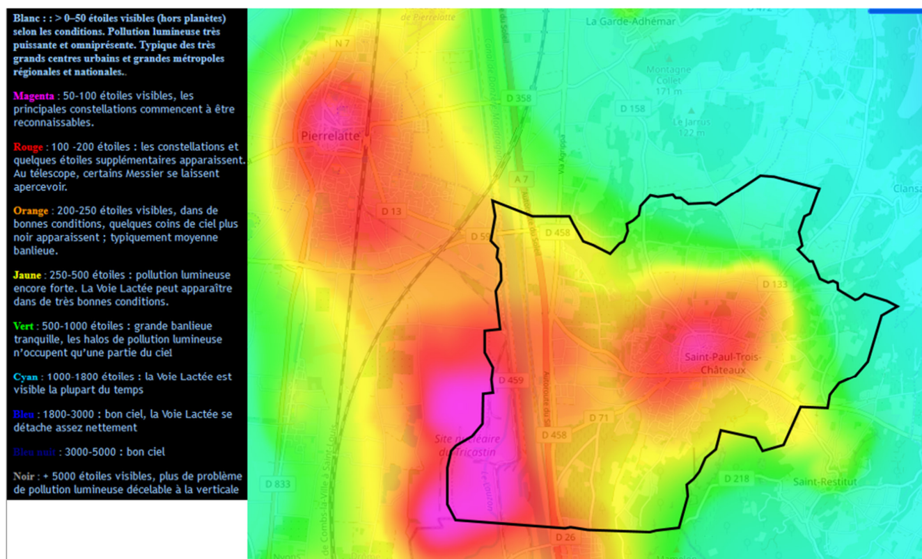
Pollution lumineuse sur le secteur – Source : Avex Asso
