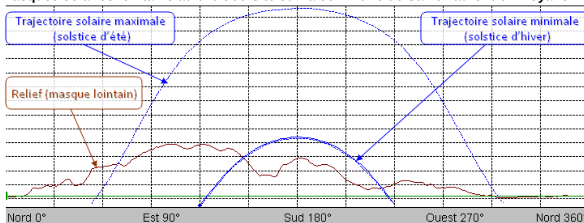
Masques solaires lointains au droit du site sur la commune de Saint-Laurent-en-Royans
