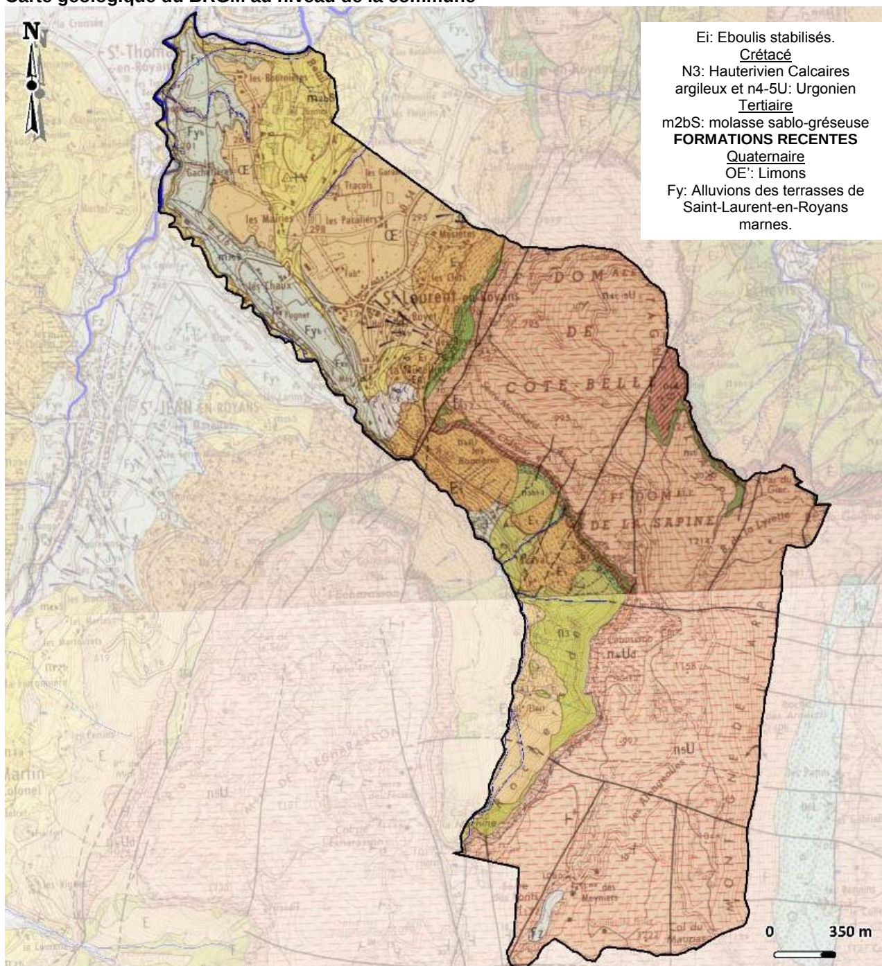
Carte géologique du BRGM au niveau de la commune
