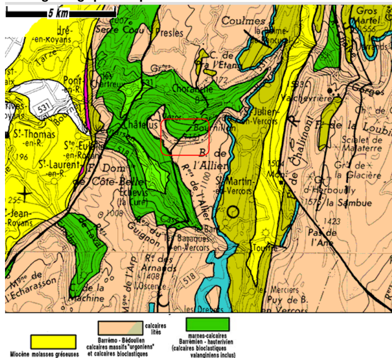
Carte géologique simplifié du secteur d'étude
