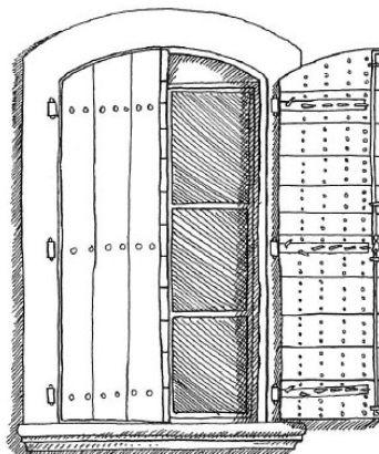
En haut : à ais contrariés, ou croisées-clouées. En bas : volets à persiennes.
