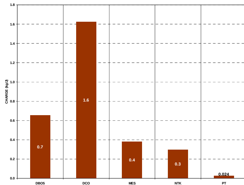
CHARGES MESUREES EN SORTIE DE FROMAGERIE
