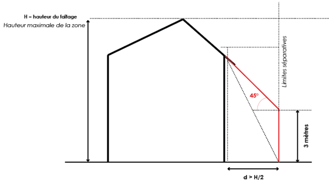
Schéma illustratif : cône de constructibilité en 1AU
