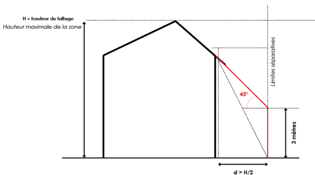
Schéma illustratif : cône de constructibilité en UA
