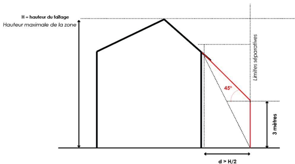
Schéma illustratif : cône de constructibilité en UB
