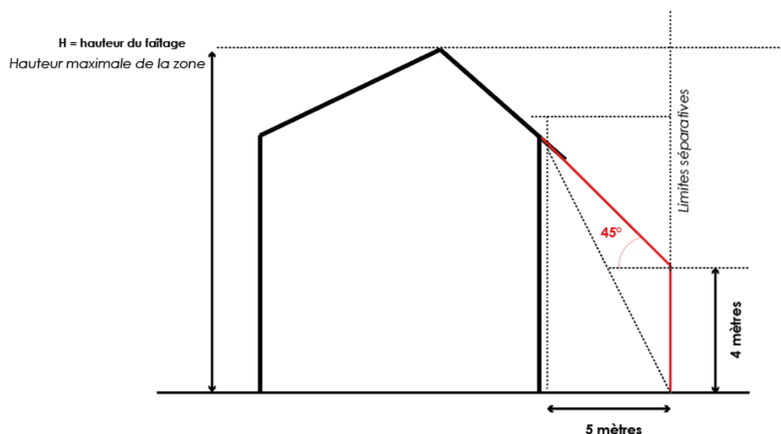
Schéma illustratif : cône de constructibilité en N
