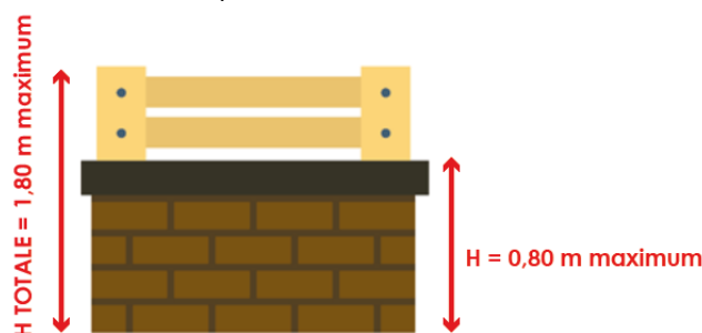
Schéma illustratif : mesure des clôtures sur limite séparative en UA
