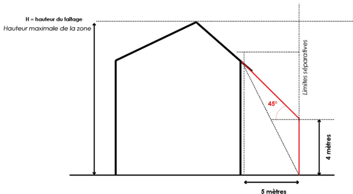
Schéma illustratif : cône de constructibilité en zone UX
