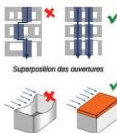
Limitation des déformations : effet «boîtes»
