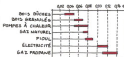
fourchettes du prix des combustibles (observés fin 2010) prix moyens TTC du kWh utile
