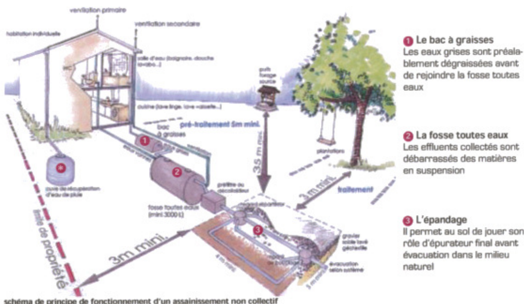
schéma de principe de fonctionnement d'un assainissement non collectif
