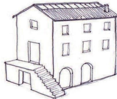
panneaux solaires en bande horizontale le long du faitage
