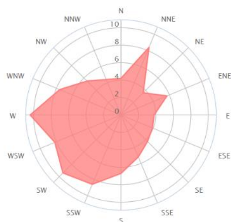
Rose des vents annuelle entre le 10/2000 et le 04/2016 à Lannion Aéroport
