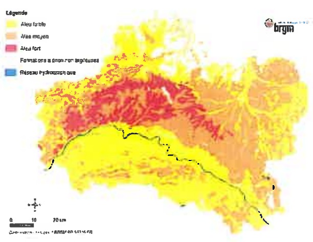
Carte d'aléa retrait-gonflement des argiles dans le département du Loiret
