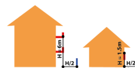
Schéma explicatif : Interprétation du recul par rapport aux baies
