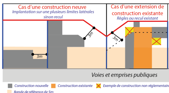
Schéma explicatif : Interprétation de la règle de recul par rapport aux limites séparatives
